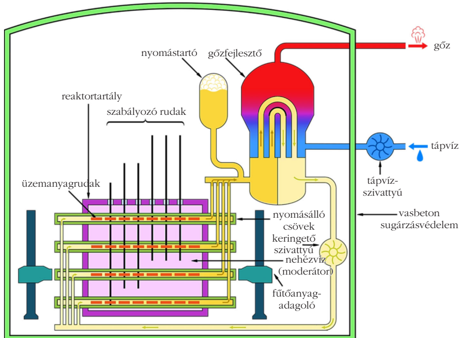
7. ábra. A nehézvízes CANDU típusú reaktor vázlata. Forrás: http://www.mvmpaks2.hu/hu/Atomenergia/AtomeromuTipusok/PublishingImages/4.%C3%A1bra.png
