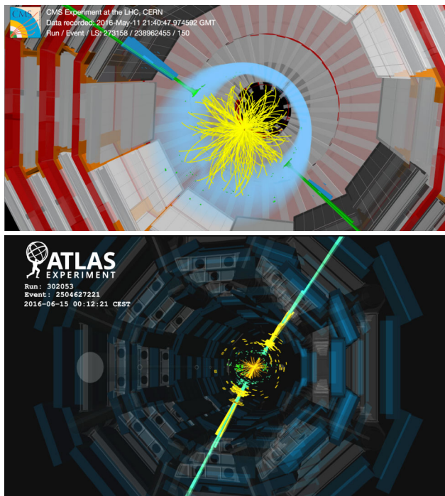
11. ábra. Óriási (6 TeV/c 2 feletti) tömegű új részecskék jelei a CMS- (föül) és ATLAS-detektorban (alul), 2016-ban. A részecskék hatalmas tömege és a belőlük felszabaduló energia mennyisége a bomlásnál létrejövő hadronzárporokat nagy mértékben fókuszálja.
