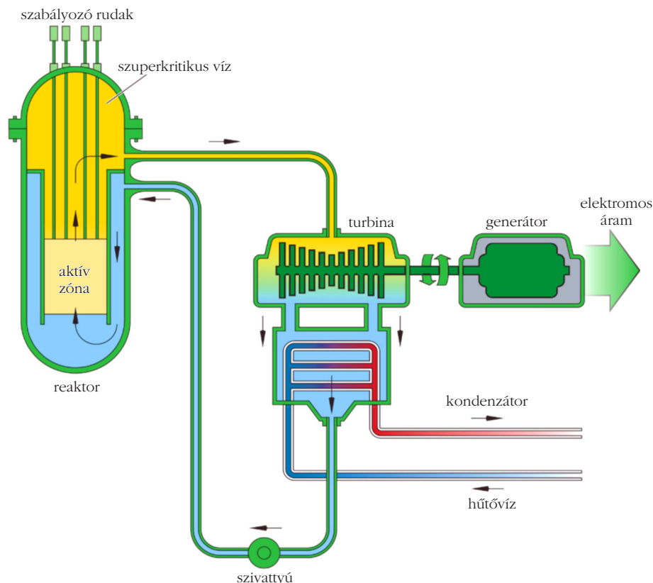
8. ábra. A szuperkritikus vízhűtésű reaktor vázlata. Forrás: http://upload.wikimedia.org/wikipedia/commons/5/59/Supercritical-Water-Cooled_Reactor.svg
