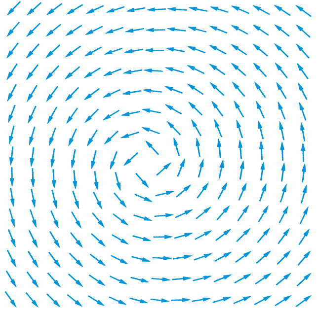
1. ábra. Vortexgerjesztés az XY-modellben, a vortexparaméter, v = 1 .
