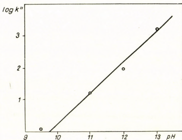
Abb. 2. Abhängigkeit des Wertes \log k'' vom pH
