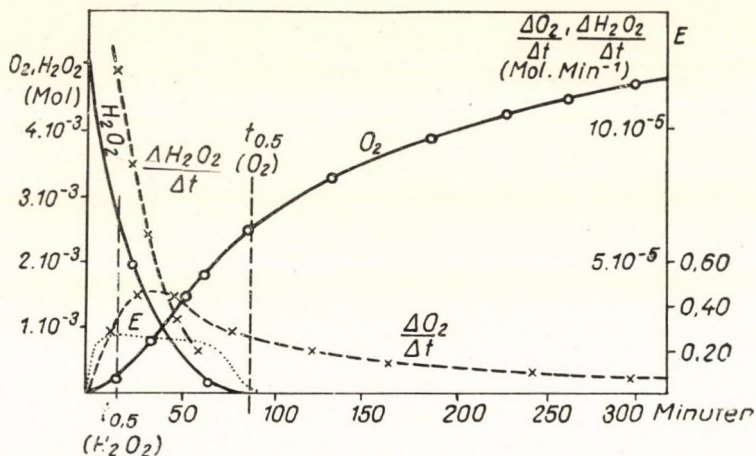
Abb. 3. Kurven der Titeränderung und der Sauerstoffentwicklung (bei pH 11) Volumen der Lösung 100 ml; 40° C; [H_2O_2]_0 = 5 \cdot 10^{-2} ; [Cu^{2+}]_0 = 2,5 \cdot 10^{-4} Mol · Liter ^{-1}
