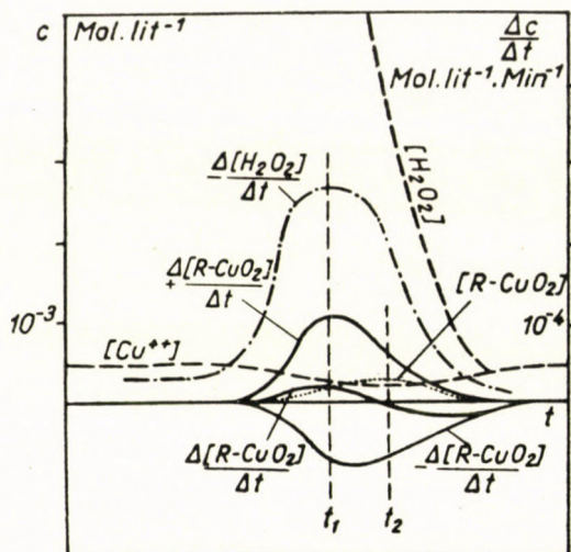
Abb. 8. Analyse der Geschwindigkeitskurven, I. [\text{H}_2\text{O}_2]_0 = 2,5 \cdot 10^{-2} ; [\text{Cu}^{2+}]_0 = 5 \cdot 10^{-4} Mol·Liter -1 ; pH 11; 20° C
