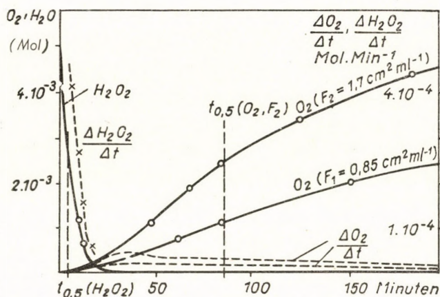
Abb. 4. Kurven der Titeränderung und der Sauerstoffentwicklung (bei pH 13) Volumen der Lösung 100 ml; 10° C; [H_2O_2]_0 = 5 \cdot 10^{-2} ; [Cu^{2+}]_0 = 10^{-5} Mol · Liter ^{-1}
