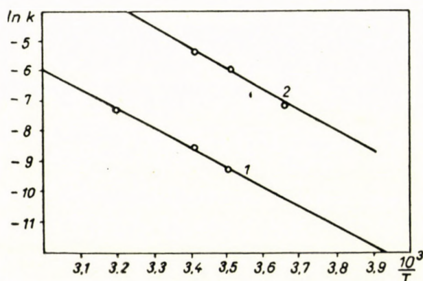
Abb. 7. 1. [\text{H}_2\text{O}_2]_0 = 5 \cdot 10^{-2} ; [\text{Cu}^{2+}]_0 = 2,5 \cdot 10^{-4} Mol · Liter -1 ; pH 11 2. [\text{H}_2\text{O}_2]_0 = 5 \cdot 10^{-2} ; [\text{Cu}^{2+}]_0 = 10^{-5} Mol · Liter -1 ; pH 13
