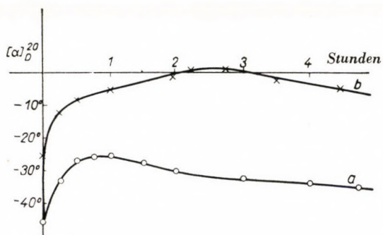
Abb. 3. Änderung der Werte von [\alpha]_D^{20} beim Kochen mit Eisessig a) im Falle reines O,N-Diacetats, b) im Falle rohes Diacetats
