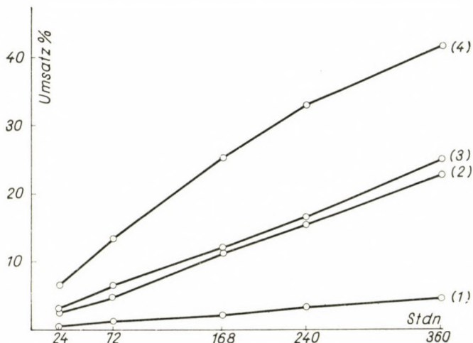
Abb. 2. N → O-Acylwanderungsgeschwindigkeit in der (±)- erythro -Reihe bei 30^{\circ} \pm 1,5^{\circ} (1) N-Benzoyl-nor-ephedrin ; (2) N-Benzoyl-ephedrin ; (3) N-Äthyl-N-benzoyl-nor-ephedrin ; (4) N-Isopropyl-N-benzoyl-nor-ephedrin
