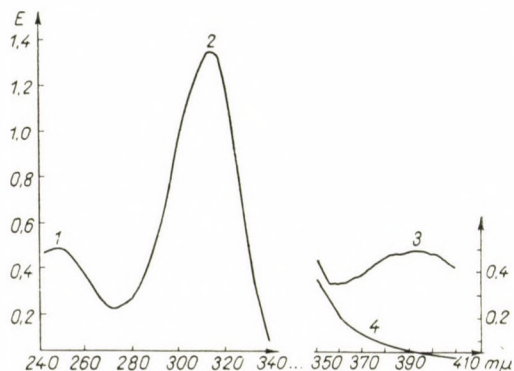
Abb. 6. Tetrabromchinon (in Chloroform) (Bromanil) ( 9,4 \cdot 10^{-4} Mol/Lit.) 1. \epsilon_{\text{max.}} : 5200, 2. \epsilon_{\text{max.}} : 14 000, 3. \epsilon_{\text{max.}} : 260, 4. Tribromphenolbrom
