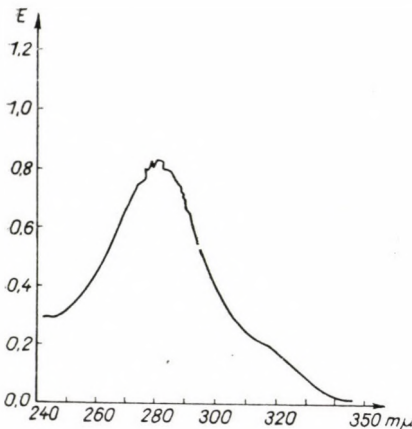
Abb. 9. Tribromphenolbrom (in Chloroform), nach Stehenlassen zwei Stunden hindurch. \epsilon_{\text{max.}} : 9000 ( 9,4 \cdot 10^{-5} Mol/Lit.)
