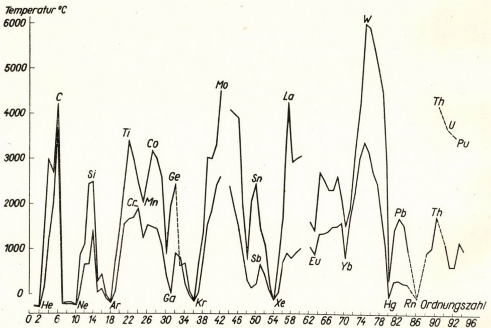
Abb. 2. Schmelzpunkte und Siedepunkte der Elemente als Funktion der Ordnungszahl
