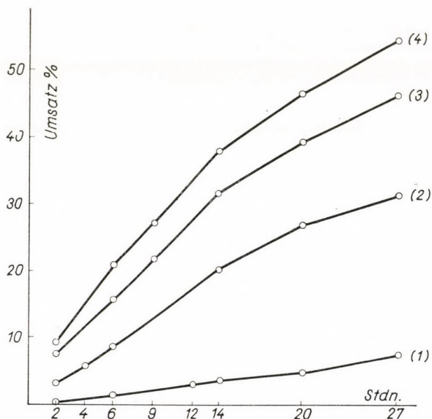
Abb. 1. N → O-Acylwanderungsgeschwindigkeit in der (±)- threo -Reihe bei 30^{\circ} \pm 0,1^{\circ} (1) N-Benzoyl- ψ -nor-ephedrin ; (2) N-Isopropyl-N-benzoyl- ψ -nor-ephedrin ; (3) N-Äthyl-N-benzoyl- ψ -nor-ephedrin ; (4) N-Benzoyl- ψ -ephedrin
