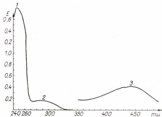
Abb. 5. p-Benzochinon (in Chloroform), 1. \epsilon_{\max} : 24 000 ( 4 \cdot 10^{-4} Mol/Lit.), 2. \epsilon_{\max} : 420 ( 4 \cdot 10^{-4} Mol/Lit.), 3. \epsilon_{\max} : 26 ( 4 \cdot 10^{-3} Mol/Lit.)
