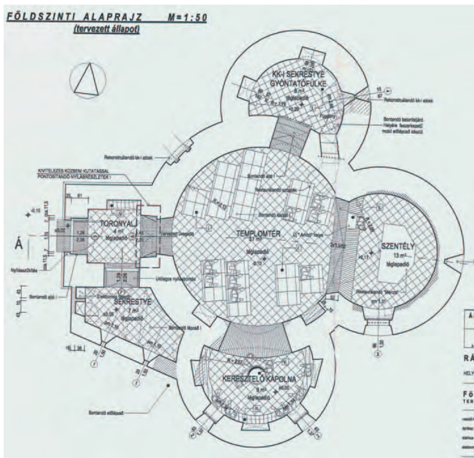
2. kép A templom tervezett alaprajza (D 3787-0001 MÉM MDK)
