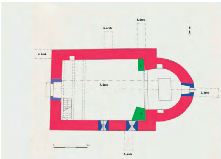
1. rajz A templom periodizációs alaprajza
