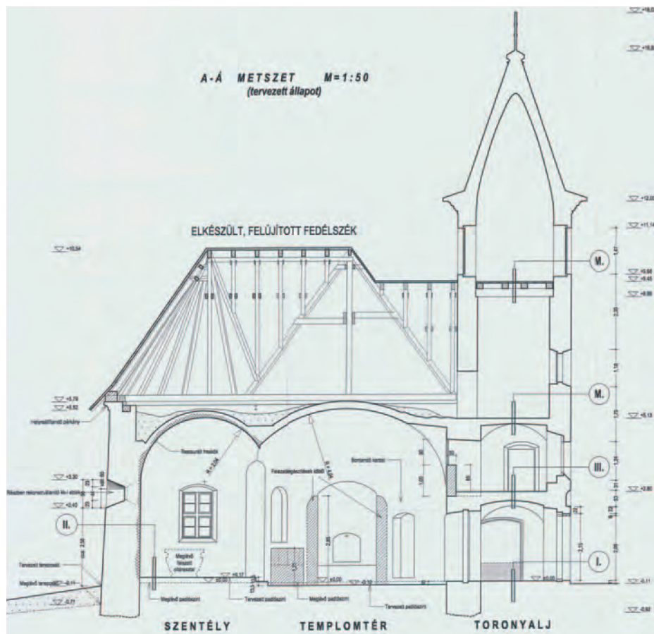
3. kép A templom tervezett metszete (D 3787-0005 MÉM MDK)
