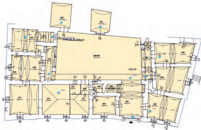
6. kép A földszint alaprajza (I-Quadrat)
