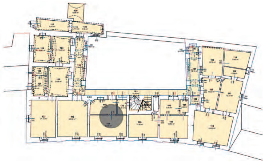
7. kép Az emelet alaprajza (I-Quadrat)
