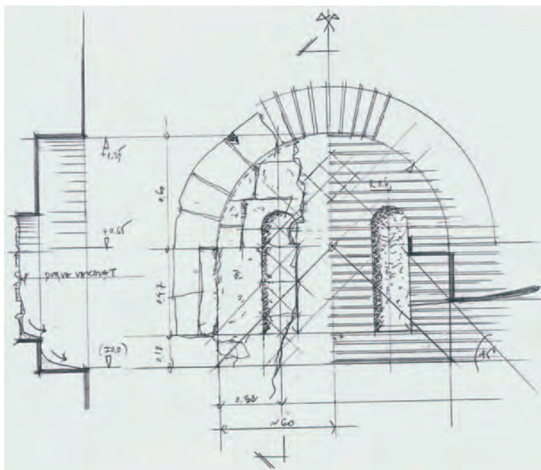
4. kép A románkori kapcsolt ablak terve (D 378870013 MÉM MDK)
