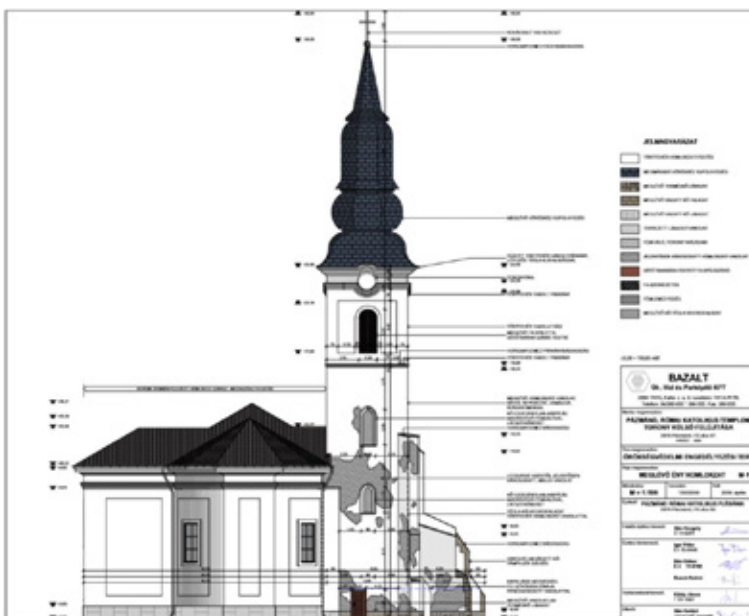
36. kép A templom északnyugati homlokzatának felmérési rajza. Bazalt Kft., 2019
