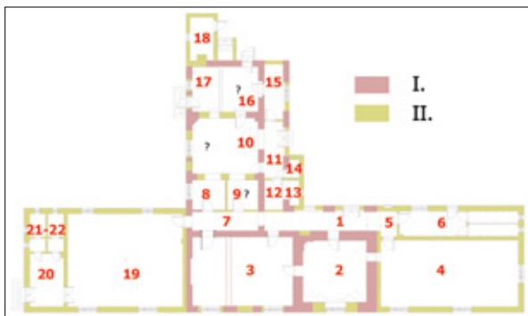
10. kép A geszti tiszttartói lak/óvoda periodizált alaprajza, a helyiségek számozásával. Az építési korszakok: I. 18. sz. közepe körül, II. 20. sz. második fele. Rajz: Design Art Werk és Mobilia Kft. felmérése nyomán a szerző
