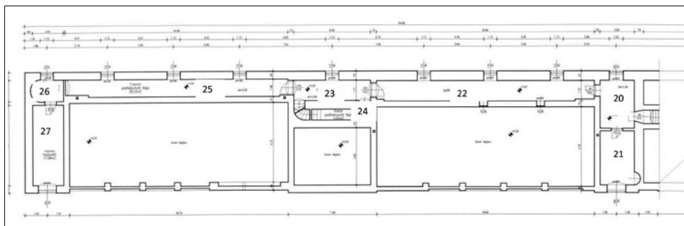
8. kép A narancsház és a kertészlak földszinti és emeleti, számozott alaprajza
