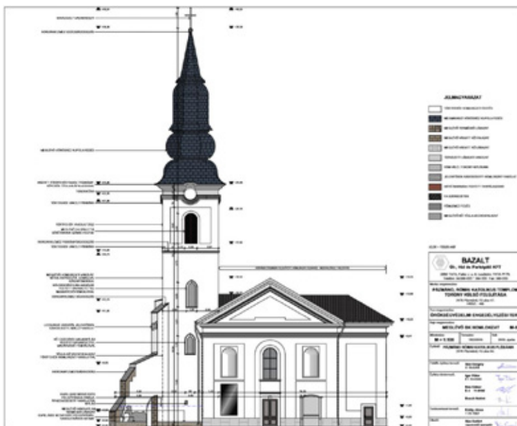
35. kép A templom délkeleti homlokzatának felmérési rajza. Bazalt Kft., 2019
