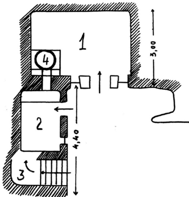
4. kép Egy régebbi típusú egerszalóki pinceház alaprajza. Bakó i. m. 1970-71. 94. kép nyomán
