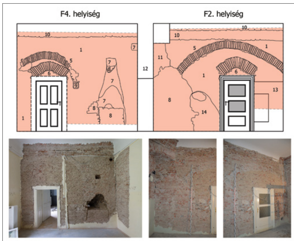
4. kép A geszti Tisza-kastély F2 és F4 helyiségeinek déli falán feltárt jelenségek. 1-téglafal, 5-elbontott boltozat lenyomata, 6-nyílás eredeti áthidalója, 7-elbontott tűzhely és szabadkémény nyomai, 8-elbontott tűzhely és szabadkémény átfalazása és fal pótlása, 9-betömött gerendalyuk, 10-falkorona magasztás, ráfalazás, 11-ismeretlen okból levéselt felület, 12-utólagos falazás, fal javítás, újrafalazás, 13-utólagos falfülke, 14-eredeti, utóbb befalazott falfülke, eredeti vakolás nyomaival. Rajz: a szerző, fotó: Bélavári Krisztina, Galamb Zsuzsanna
