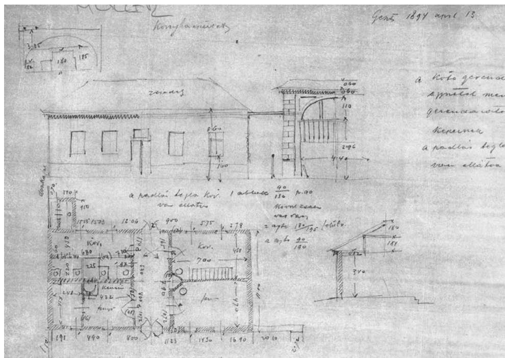
6. kép Möller István felmérése a geszti Istálló nyugati szélén álló lakóházról, alaprajz és metszet, 1894.
