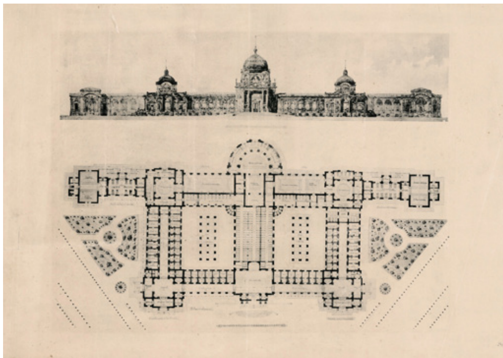
12. kép Czigler Győző–Dvořák Ede–Gerster Kálmán: a városligeti Széchenyi fürdő alaprajza és homlokzatterve, 1908 körül, tervfotó MÉM MDK Magyar Építészeti Múzeum ltsz.: 80.01.75
