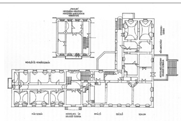
12. kép A kastély rekonstruált elrendezése
