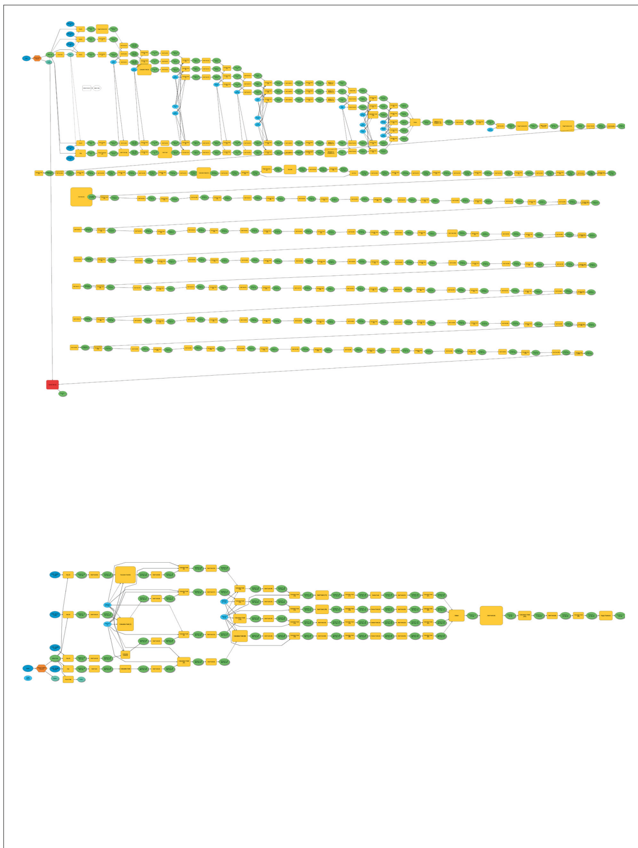
3. ábra: A CLC100-as adatbázis feldolgozásának folyamata ArcGIS ModelBuilderben 4. ábra: A CLC100-as változásadatbázis feldolgozásának folyamata ArcGISModelBuilderben
