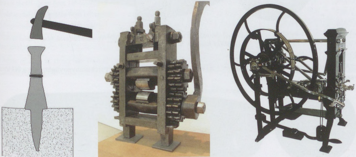
11. ábra Kézi verés, pofás verőgép, Uhlhorn-féle verőgép
