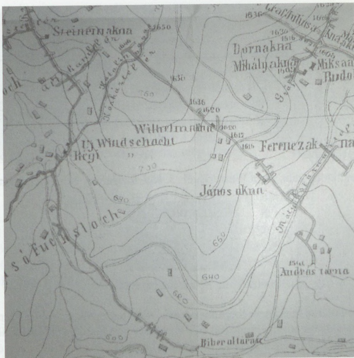
3. kép. Az András-tárna és a Katalin-vágat helyzete 1646–1648-ban
