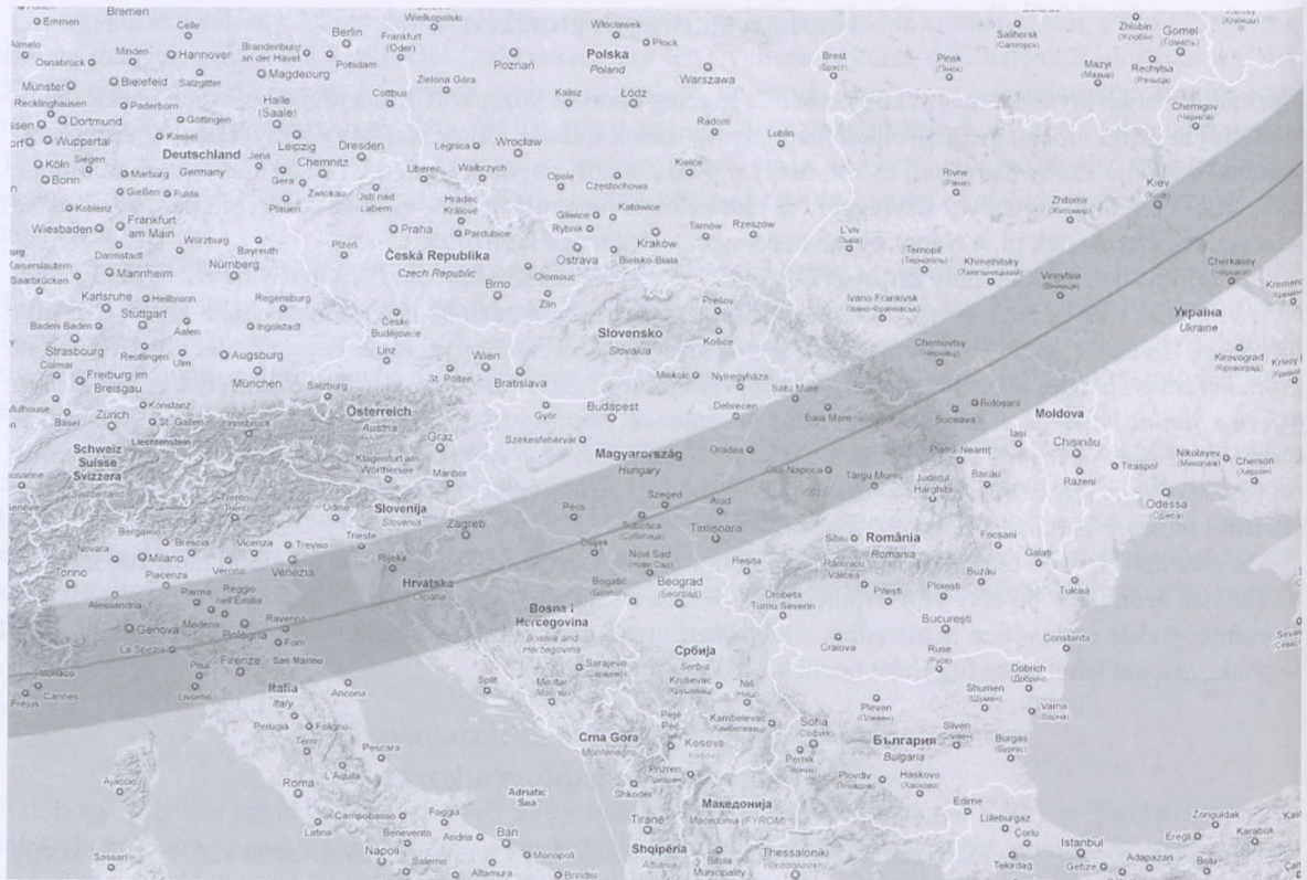
Az 1270. március 23-i napfogyatkozás legnagyobb (99%-os) sávja
