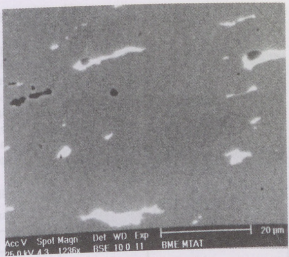
5. kép 2. BRBAJ9301 1236× (EDS) Fehér alapon szürke (Ag) foltok
