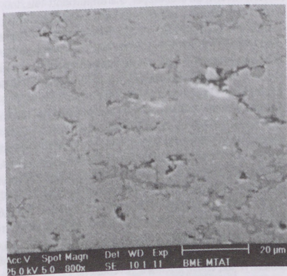
6. kép 4. BRBAJ9602 800× (EDS) Fekete (Fe) foltok a pénz alapanyagában
