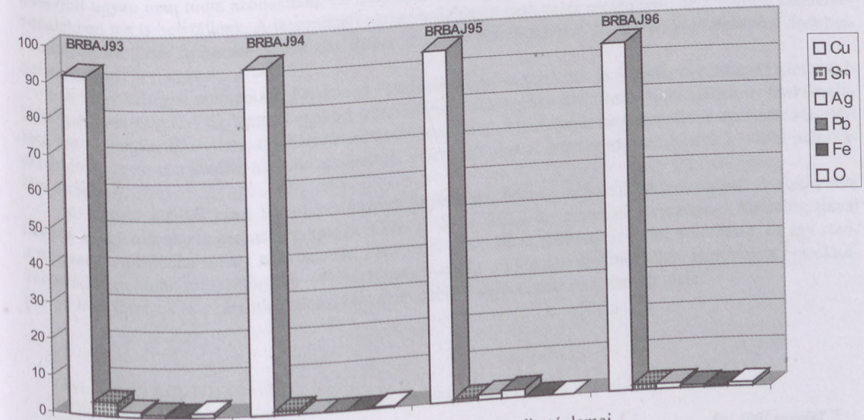
7. kép Késő római rézpénzek fő alkotóelemei
