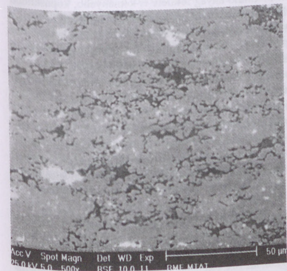
6. kép 3. BRBAJ9402 500× (EDS) Pénz oxidálódott alapanyaga
