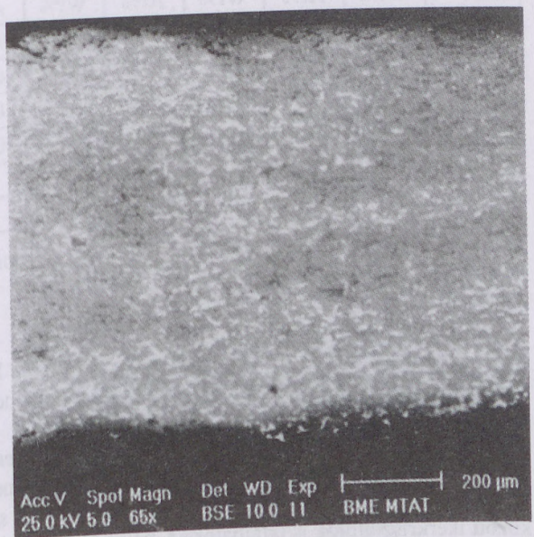
5. kép 4. BRBAJ9401 65× (EDS) Pénz alapanyaga
