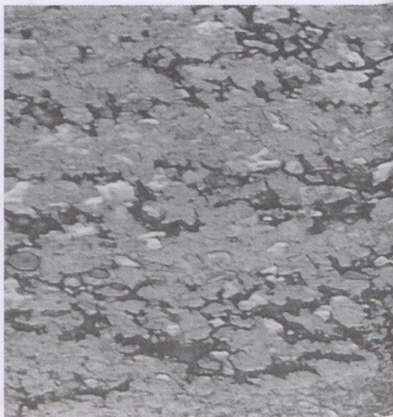
4. kép 2. BRBAJ96e 400× Érme húrirányú metszete, részlet, a belső részeken laza, az élek irányába elnyújtott szövetszerkezettel
