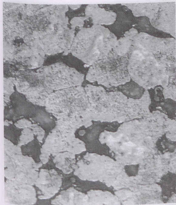
2. kép 1. BRBAJ93f 400× Érme hűrirányú metszete, részlet, a belső részekben teljesen laza szövetszerkezettel
