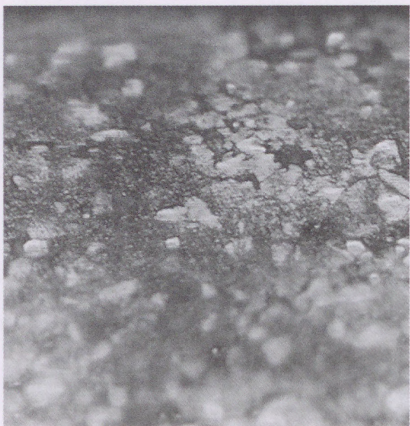
4. kép 1. BRBAJ96d 400× Érme húrirányú metszete, részlet, a felszín közelében teljesen tömörödött szövetszerkezettel
