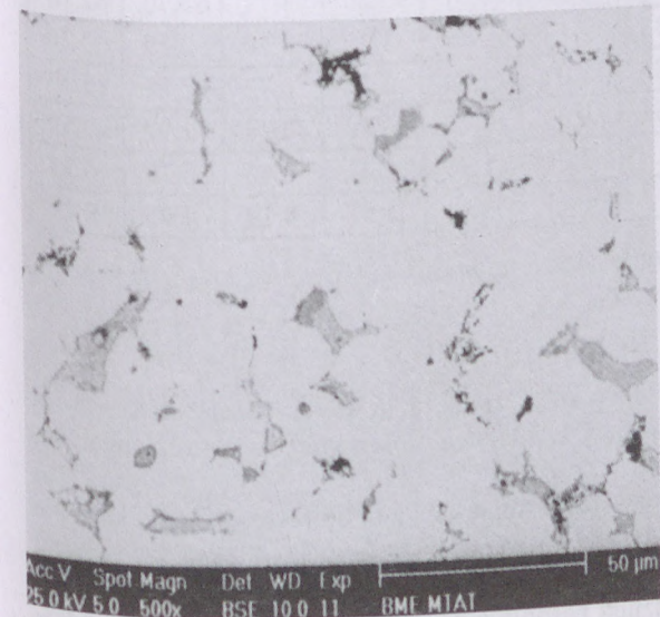
5. kép 3. BRBAJ9302 500× (EDS) Pénz alapanyagában fehér (Pb) foltok
