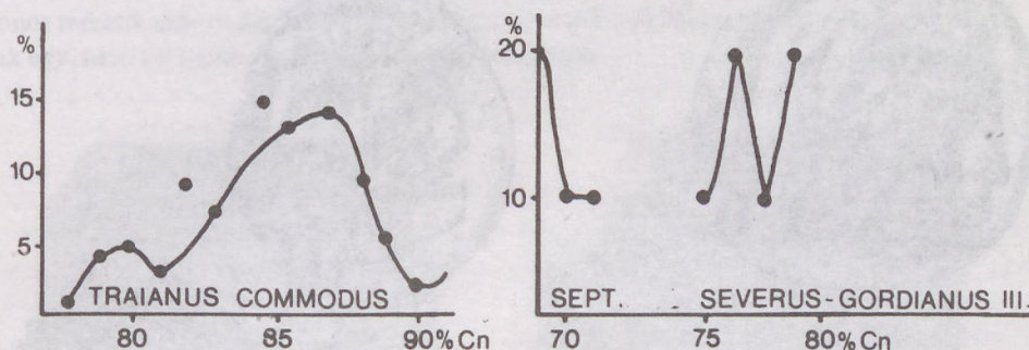
4. ábra Sestertiusok Cu tartalom eloszlásának gyakorisági görbéi
