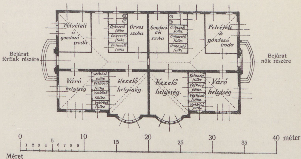
Alaprajz.
