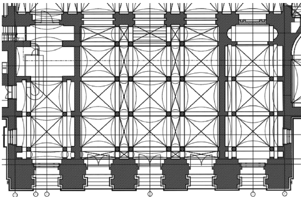
3. kép A Diszterem alatti földem tartószerkezeteinek alaprajzi elrendezése. (Forrás: Közti Zrt.)
