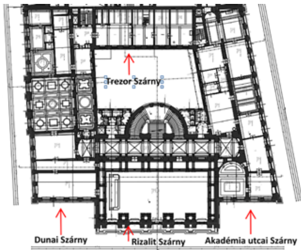
1. kép MTA Székház –Alaprajzi elrendezés. (Forrás: Közti Zrt.)
