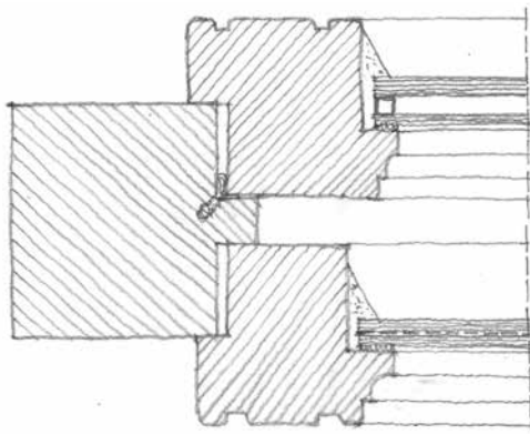
5. ábra Első javaslat az ablak teljesítménynövelő felújítására. A külső szárnyban vékony szigetelő üveg, a belsőben zajvédő laminált üvegtábla.
