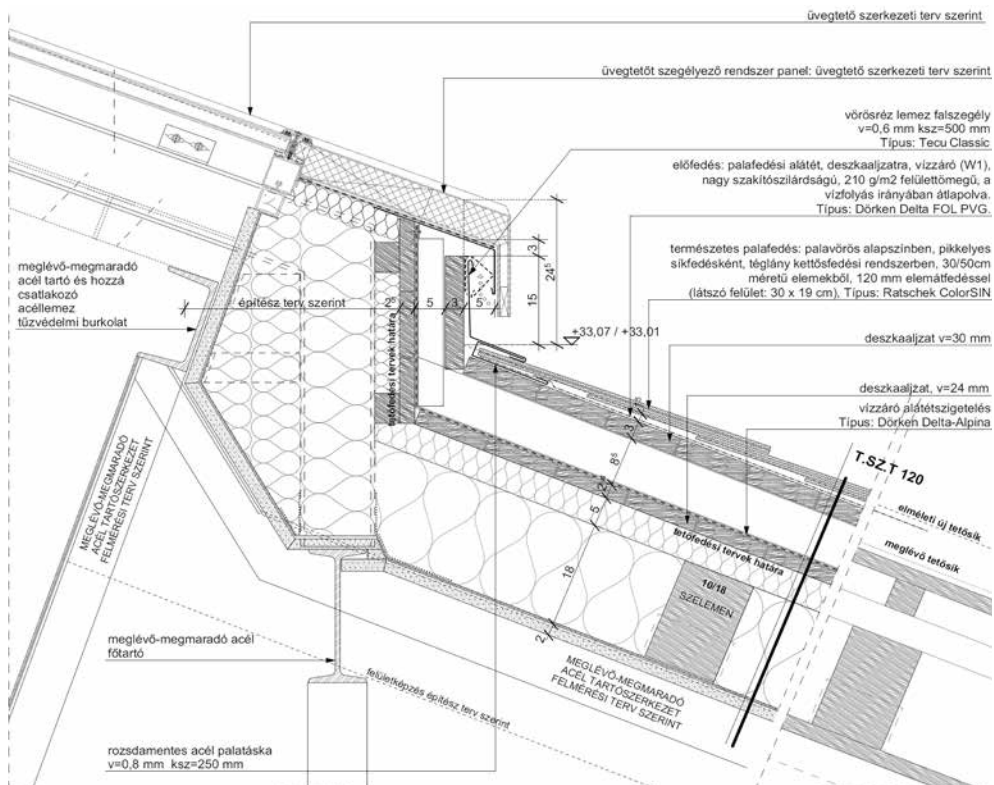
4. kép Az üvegeltető csatlakozásának terve, a tető kiszellőzését is lehetővé tevő kialakítással.
