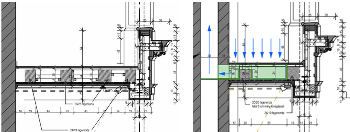
6. kép Karzati metszetek (Forrás: Közti Zrt.)
