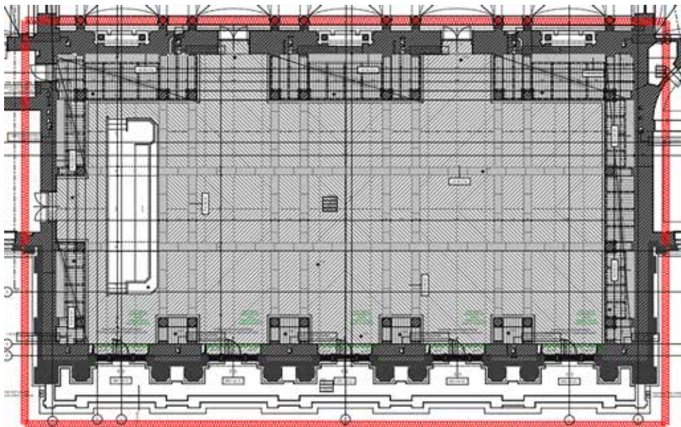
4. kép Diszterem – első emeleti alaprajzi elrendezés. (Forrás: Közti Zrt.)
