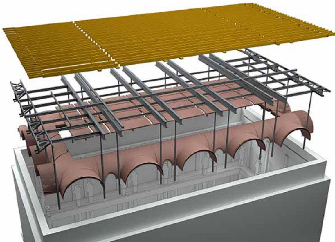
7. kép A Díszterem feletti kettős földem szerkezete felújítás előtt. (Forrás: Paulinyi & Partners Zrt.)
