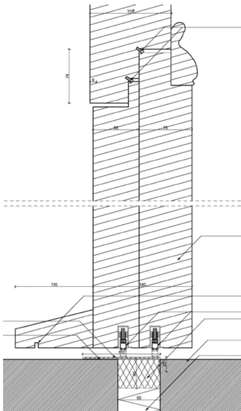
7. ábra A loggiára vezető ajtó tervezett tömítései a kiviteli tervben.
