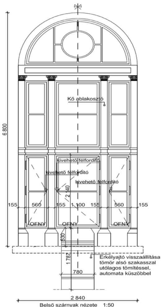
1. ábra Egy ablak a kiviteli terv konszignációs lapján.
