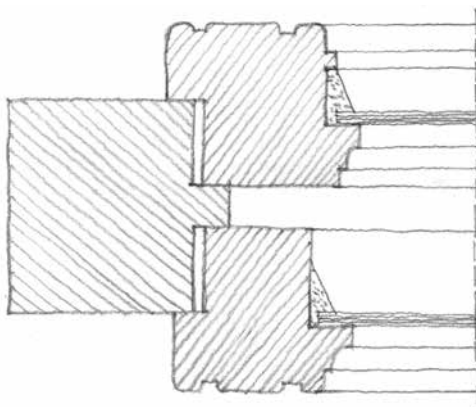
2. ábra Az ablak felmérési metszeti részlete. A belső szárny formája ekkor még feltételezés a rá csavarozott ideiglenes vendégszárny miatt.
