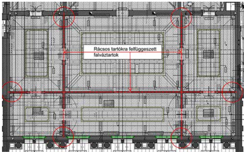
10. kép A Díszterem feletti képtár függesztett válaszfalainak tartószerkezeti elrendezése. (Forrás: Közti Zrt.)
