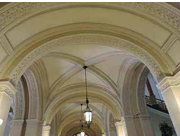
2. kép – Díszterem alatti födém csehsüveg boltozata és a boltmezőket szegélyező hevederívek – részlet. (Forrás: Általános tartószerkezeti szakvélemény - Közti Zrt. és Baratta Építész és Mérnöki Iroda Kft.)
