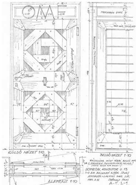
15. kép Az első emeleti bejárati ajtó 1984-es, Sedlmayr János által rajzolt, 1:10 léptékű terve. (Forrás: Sedlmayr-Nagypál 1981)
