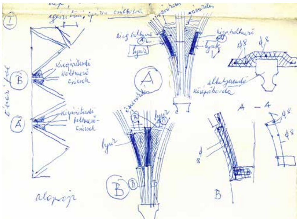
8. kép Sedlmayr János levélmellékleteként a kivitelezőnek megküldött vázlata (1976. január 6.) a vasbeton héjak kialakításával kapcsolatban. (Forrás: Győr-Moson-Sopron Vármegyei Kormányhivatal Építésügyi és Örökségvédelmi Főosztály tervtára)
