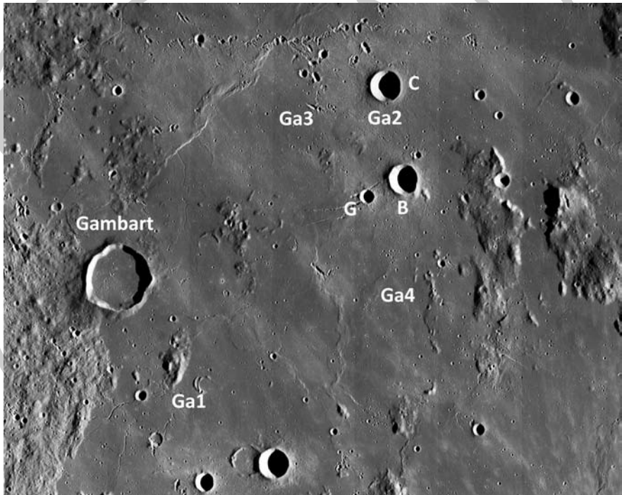
A Gambart-kráter és a dómkok az LRO (Lunar Reconnaissance Orbiter) nagymozsaikjából kivágott részleten (NASA)
