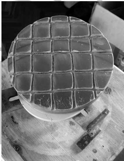
A képen az alumínium hordozóra öntött szurok. Akkor megfelelő, ha félórányi munka után láthatóan szűkülnek a bevágott csatornák, pár óra után pedig újrávágás szükséges. Mint ebben az esetben is.
