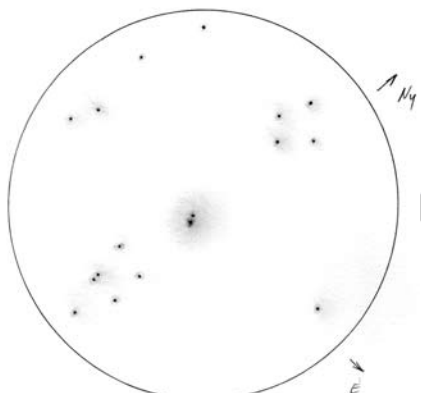
Az \alpha CVn Talabér Gergely rajzán (2021. március 31., 9 L, 46x, PA 230)
