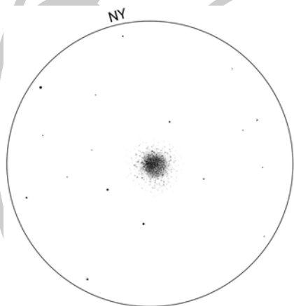
Domán Tamás 2021. június 6-án észlelte az M3-at. 12,7 MC: 46x-os nagyítás is bontotta, de igazán szép látványt a 17 mm-es (88x) okulárban mutatott, ahol már határozottan csillagaira bomlott a halmaz
