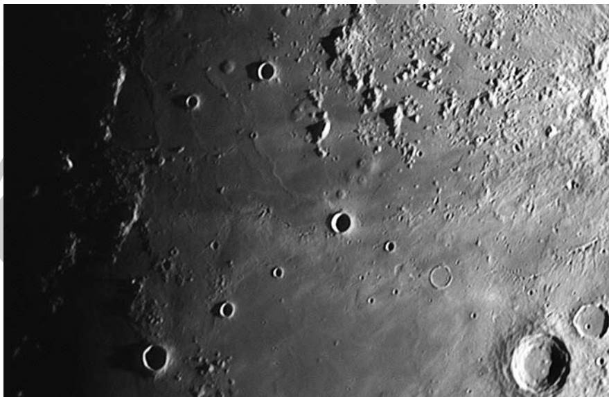
Kocsis Antal szakszoportvezető a Balaton Csillagvizsgáló 304 mm-es f/10-es Meade SC teleszkópjával és DMK41 AU02.AS kamerával készítette ezt a felvételt, amelyen kiválóan láthatóak a Hortensius-dómkok. A felvétel 2014. július 7-én készült
