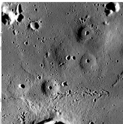
A Hortensius-dómkok az LRO (Lunar Reconnaissance Orbiter) nagy felbontású felvételén
