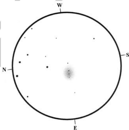
Az NGC 6846 (355/1650 T, 413 \times , 4 ívpercnyi részletrajz)
