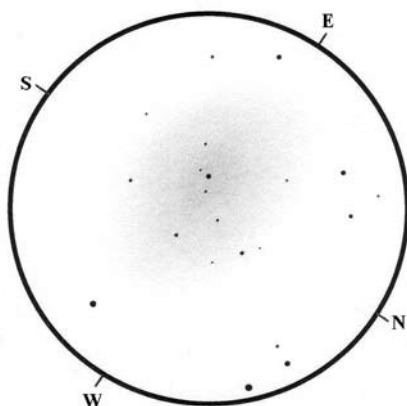
Az IC 166 (355/1650 T, 275×, 7 ívpercnnyi részletrajz)
