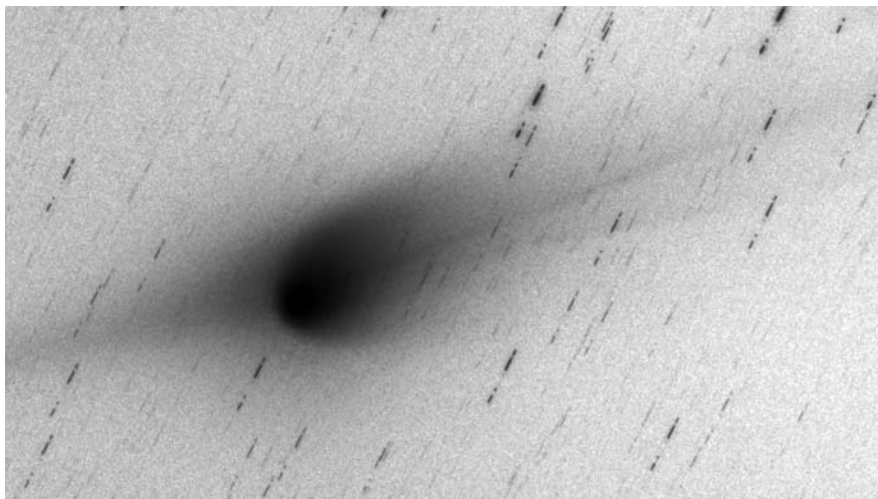
Jobban megnézve Sebestyén Attila 2023. január 23-án 1:23 UT-kor készült képét, jól látszik, hogy az ellencsóva látszólagos. Valójában a csóvára látunk rá felülről, de nagyon lapos szögben. (150/518 T + Player One Uranus C; Gain: 300; 25x60 s)
