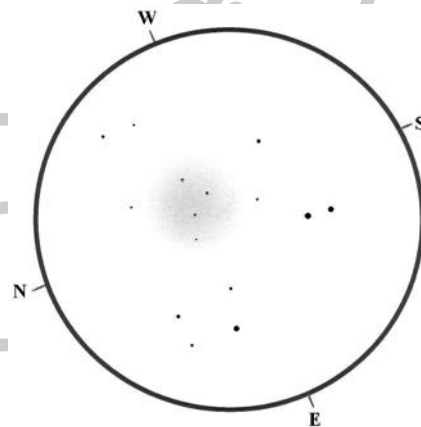
A Saurer 6 (355/1650 T, 275x, 5 ívpercnyi részletrajz)
