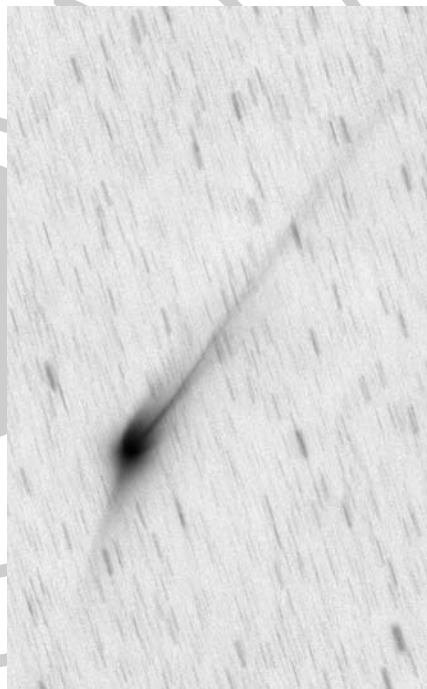
Balázs Gábor szép felvétele a „háromcsóvás” üstököséről 2023. január 25-én 00:32 UT-kor. (135 mm teleobjektív + EOS 250D; ISO 800; 35x120 s)
