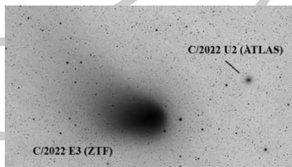
Többen kísérleteztek az üstökös-együttlés megörökítésével 2023. február 6-án. Ezek közül most Majzik Lionel fotóját mutatjuk be. (80/400 L + ASI 183MM Pro; Gain: 111; 120x30 s)
