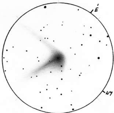
Az üstökös vizuálisan is szép látványt nyújtott például Rotaru Benjamin Daniel 254/1200 Newton távcsövében 67x-es nagyítást használva 2023. január 30-án 00:50 UT-kor (a látómező 45 ívperc átmérőjű)
