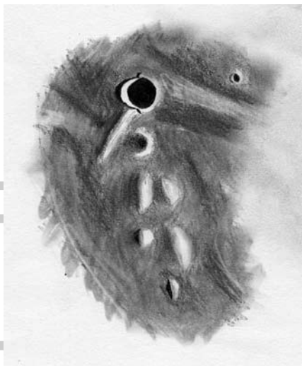
A Hortensius és dómjai 2022. április 11-én, Kárpáti Ádám rajzán (100/1000-es TAL-refraktor, 167x-es nagyítás, zenittűköt)
