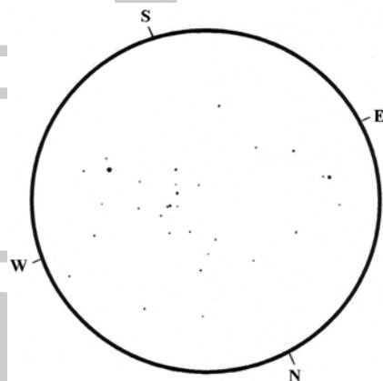
Az NGC 7067 (254/1200 T, 300x, 5 ívpercnyi részletrajz. A rajzokat a szerző készítette)
