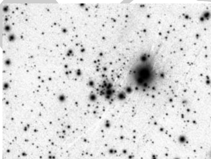
A Kumar 21 nyílthalmaz a PanSTARRS felvételén. A fotón legfényesebben ragyogó csillag a szövegben említett kettős 11 magnitúdós komponense
