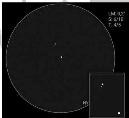
Domán Tamás rajza a 40 Eridanin ábrázolja. A kép jobb alsó sarkában láthatjuk a kinagyított rendszert
