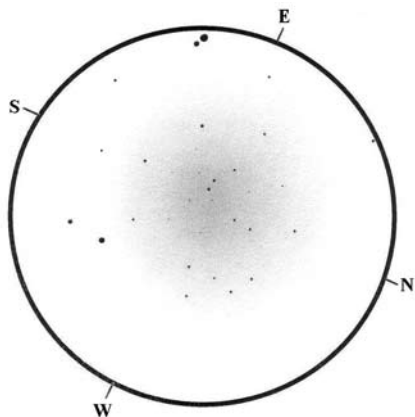
Az NGC 609 (355/1650 T, 413×, 5 ívpercnnyi részletrajz)
