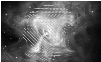
A 6500 fényévre levő Rák-ködben levő pulzárt körülvevő bonyolult ködösség. A ködösség képét a Hubble-űrtávcső, valamint a Chandra röntgentávcső felvételeiből állították össze, míg a mágneses tér vonalakkal jelzett irányára vonatkozó adatokat az IXPE szonda szolgáltatta (NASA/Bucciantini et al.; NASA/CXC/SAO; NASA/STScI; NASA-JPL-Caltech)
