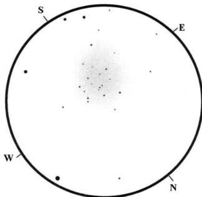
Az NGC 136 (355/1650 T, 550x, 4 ívpercnyi részletrajz)
