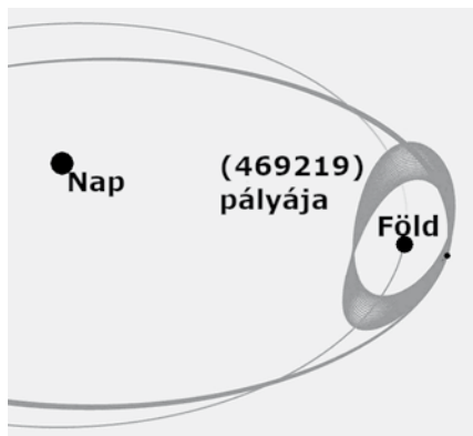
A (469219) Kamoʻoalewa kisbolygó a 2023 FW13-éhoz hasonló pályája, amely révén a Földdel rezonanciában keringve a Nap körül bolygónk kváziholdjának tekinthető (NASA / JPL-Caltech)
