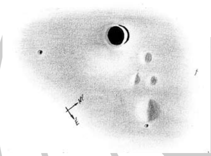
A Hortensius-kráter és a tőle északra fekvő dómok Horváth László István 2006. április 8-án készült rajzán. 11,4 T, 150x
