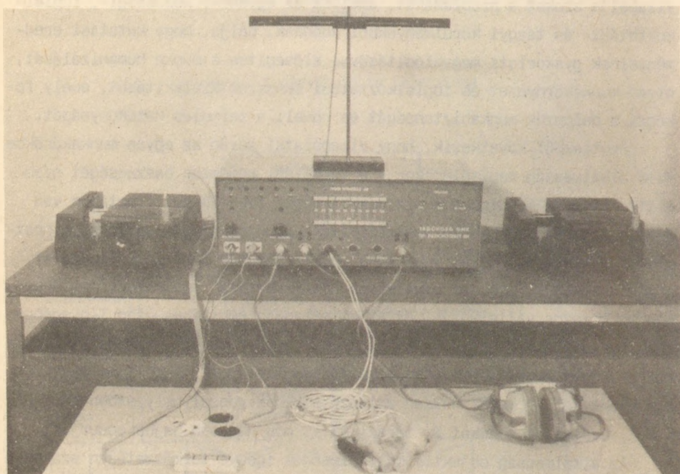
4. ábra: Számítógéphez on-line kapcsolt szívritmus-, bőrellenállás-, reakcióidő és kettős tachiszto-projektor PSZICHOTESZT-101 pszichológiai mérőrendszer
