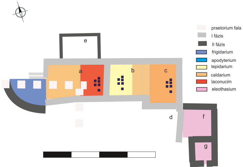
4. ábra. Vármező (Buciumi) tiszti fürdő, melyben a – caldarium/laconicum (?), b – tepidarium/caldarium (?), c – tepidarium (?), d – frigidarium/apodyterium (?), apszis-frigidarium (?)
