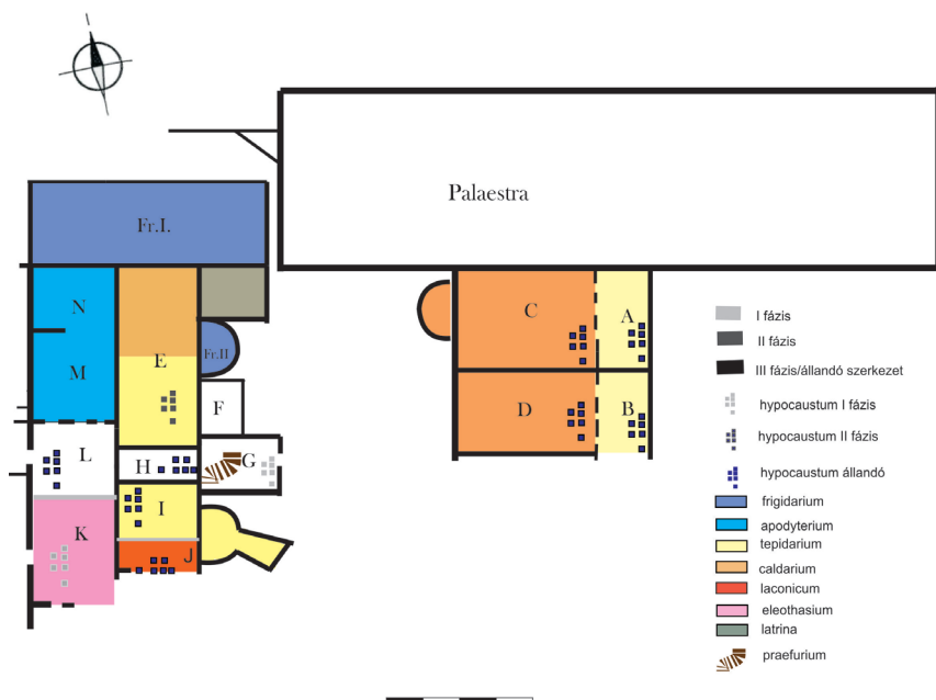
1. ábra. Potaissa (Torda/Turda) fürdő, melyben A–B – tepidárium (?), C–D – caldarium (?), E – tepidarium/caldarium (?), G – praefurnium, I–J – apszis – caldarium/laconicum (?), K – eleothesium (?), M–N – apodyterium (?), P – palaestra, Fr.I. – frigidarium, Fr.II. – frigidarium, ? – latrina, F–H–L – nem tudni
