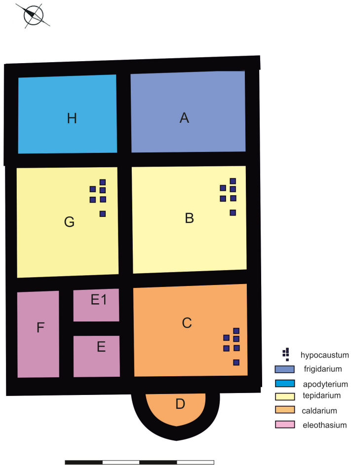
2. ábra. Resculum (Sebesvár/Bologa) fürdő, melyben A – frigidarium, B – tepidarium, C – caldarium/laconicum (?), D – medence, feltehetően caldarium (?), F-E1-E – eleothesium (?), G – tepidarium (?), H – apodyterium
