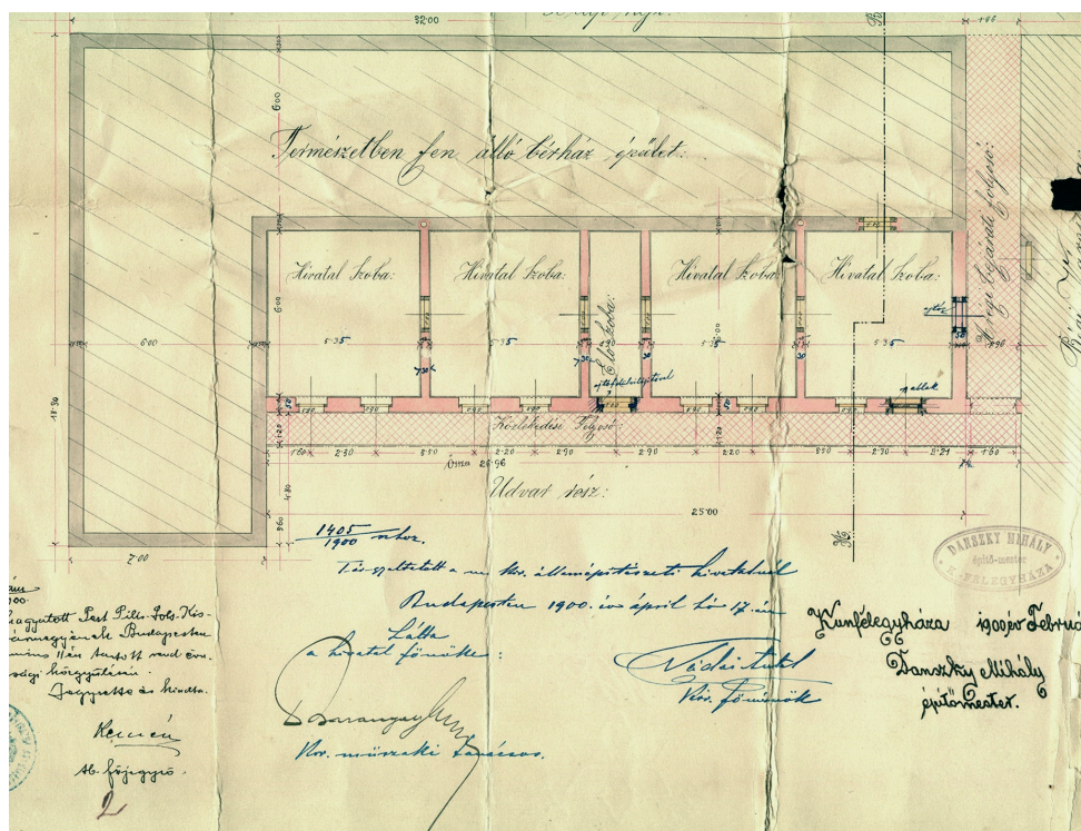
A Bazár-épület hivatali helyiségekkel kibővített, udvari részének alaprajza (HU-MNL-BKML-V.175.b. 2768/1899)
