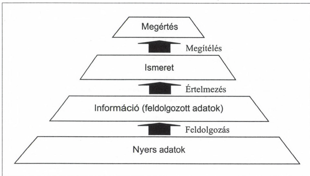
1. ábra. Információ-hierarchia.
