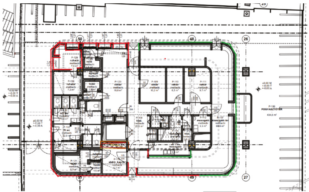
18. A Déli pályaudvari felvételi épület Bisztró alaprajza (az utascsarnok részlete). Markó András, MÁV Beruházás Lebonyolító Igazgatóság, Műszaki Tervezési Osztály, 2023. Piros színnel jelezve a murália megmaradt, zölddel a rekonstruálandó szakaszai. (Branczik Márta, 2023)
