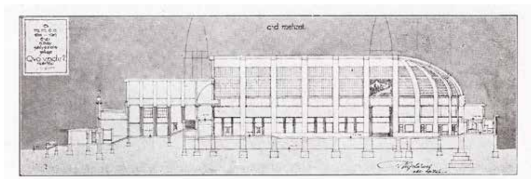
14./b. Kiss László: Jégpalota pályázati terve, hosszmetset, 1911
