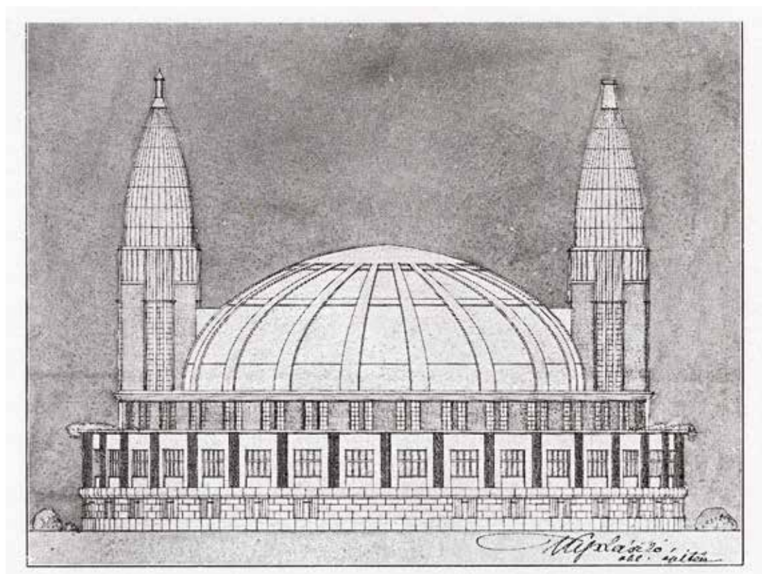
14./a. Kiss László: Jégpalota pályázati terve, hátsó homlokzat, 1911
