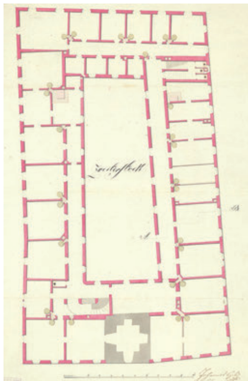
9. Második emeleti alaprajz. Hild János, 1807/1811
