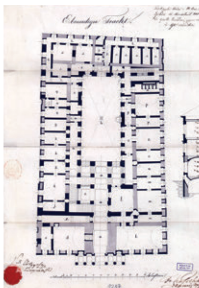
10. Kasselik Ferenc terve a városháza földszintjéhez, 1842 (?)
