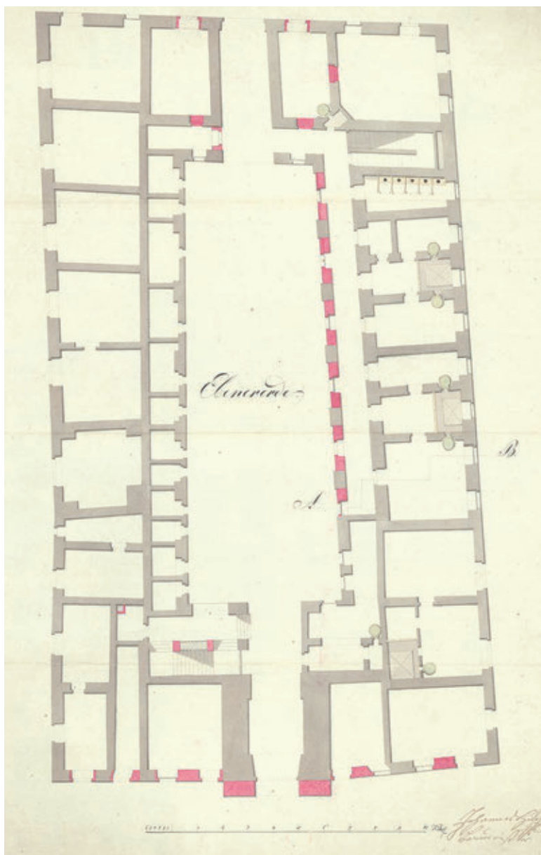
7. Földszinti alaprajz. Hild János, 1807/1811
