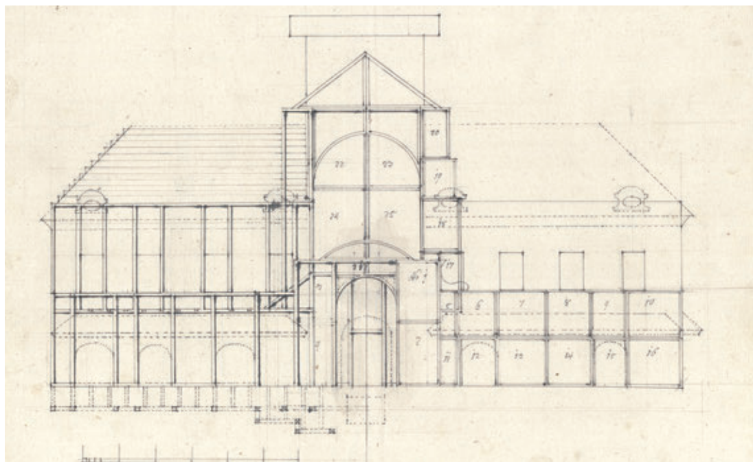
6/b. A vázszerkezet terve, 1790
