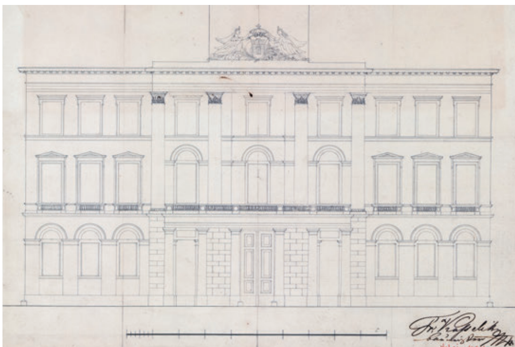
7. Kasselik Ferenc terve az új városháza főhomlokzatához, 1837 (?)
