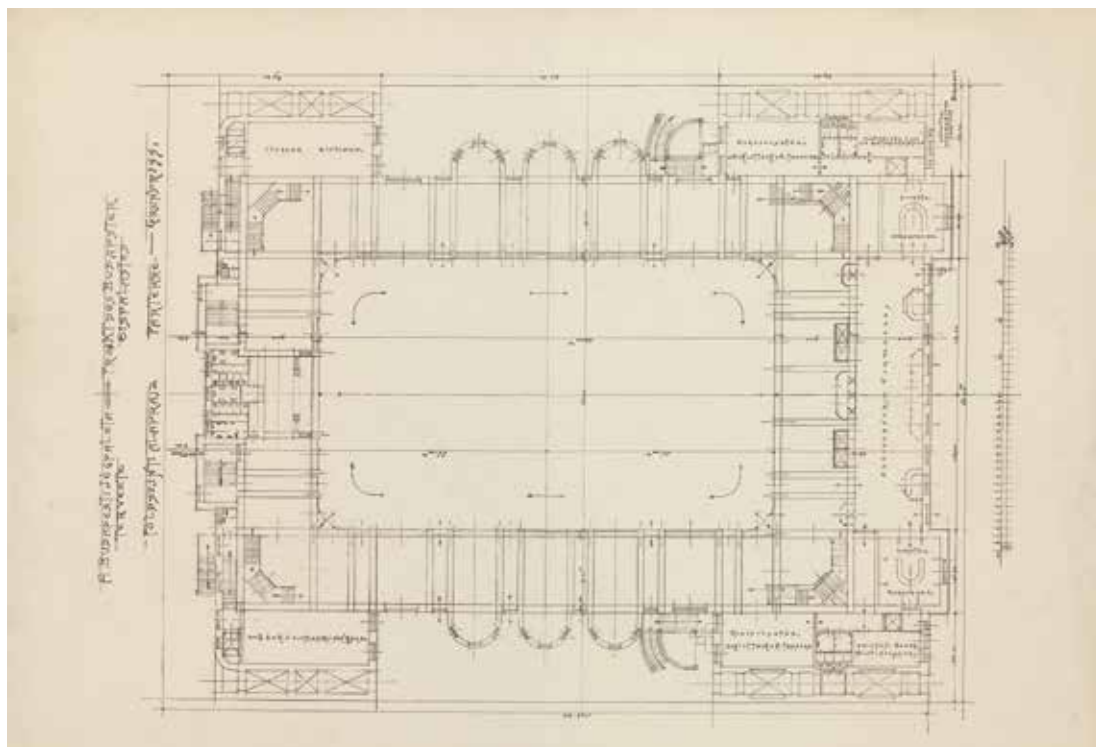
4. Mayer Péter: Jégpalota terve, földszinti alaprajz, 1909
