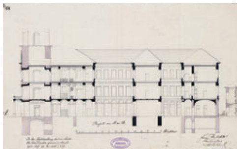
3. Kassalik Ferenc metszeti terve az új városházához, 1837 (jobbra a régi részlete)
