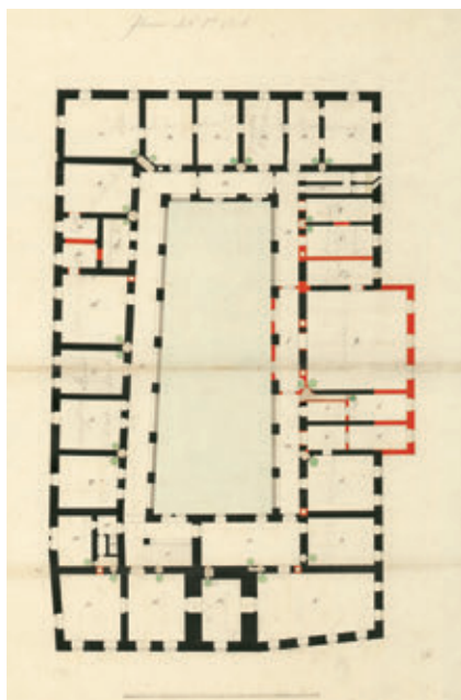
13. Emeleti alaprajz változata. Zitterbarth Mátyás, 1821
