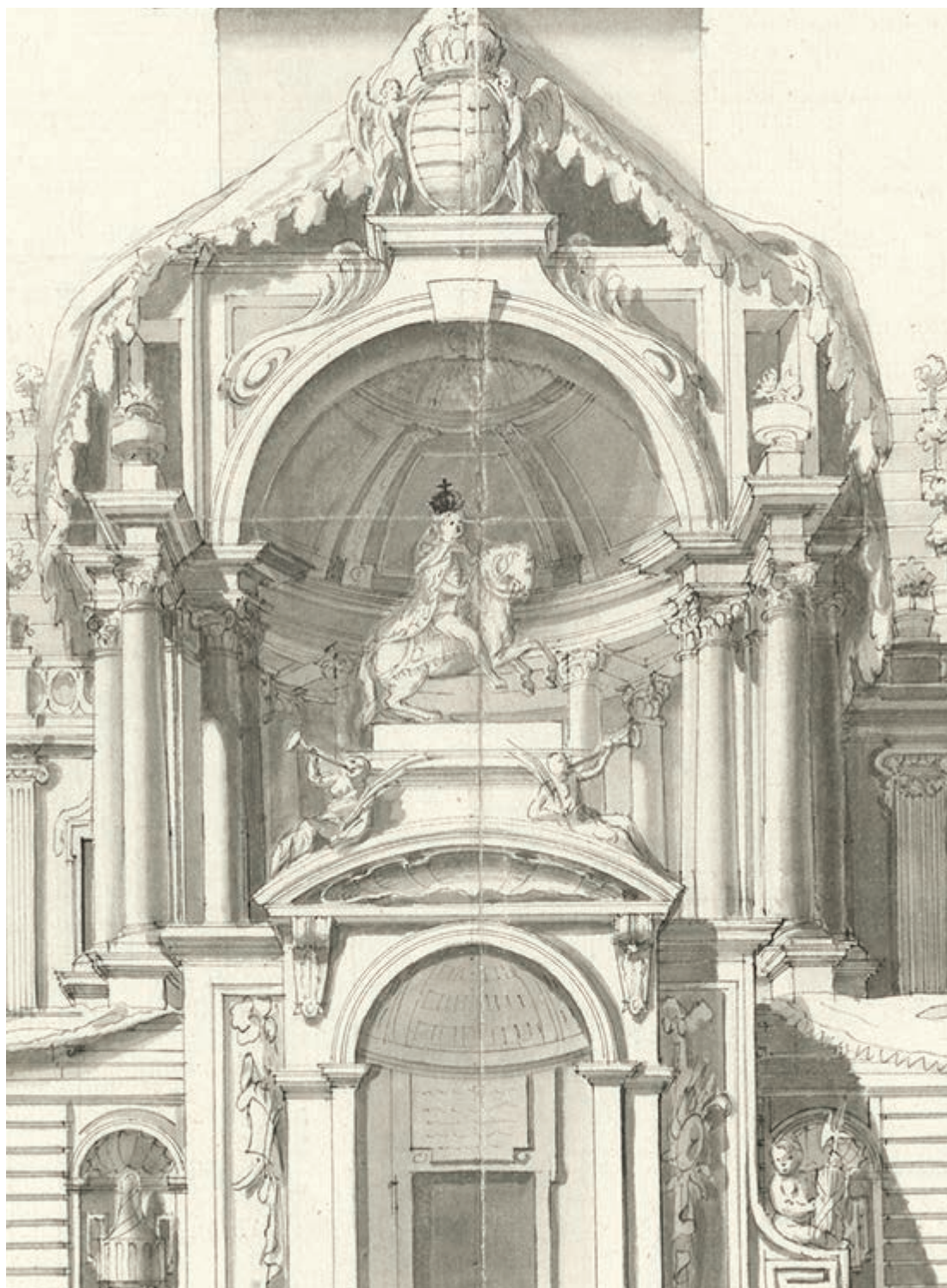
A II. Lipót koronázása alkalmából a városháza előtt felállítandó díszépítmény terve (részlet)
