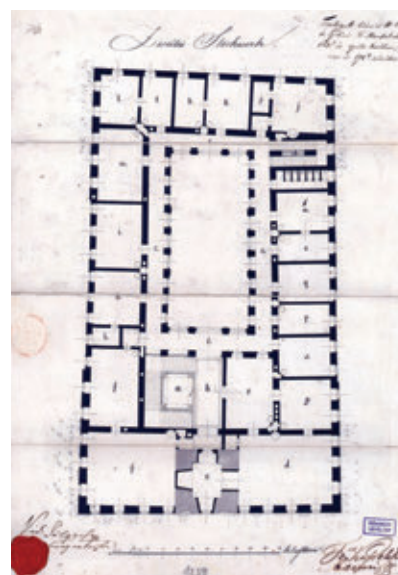
12. Kasselik Ferenc terve a városháza második emeletéhez, 1842 (?)
