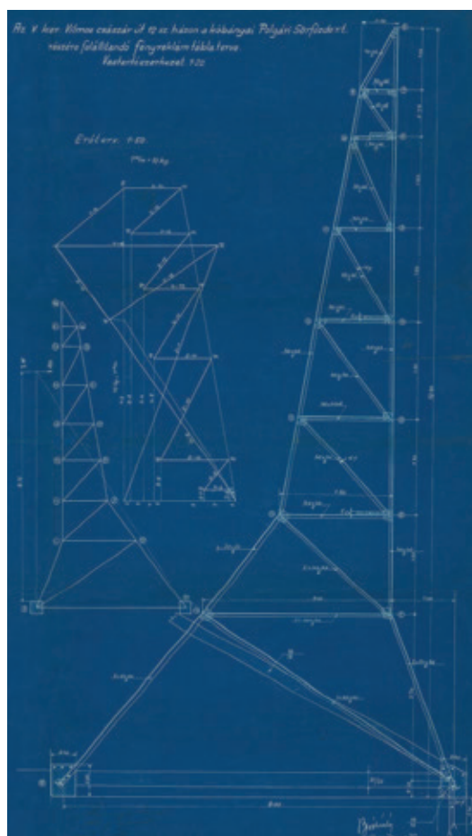
2. Vilmos császár út 12., a vastartószerkezet tervrajza, 1925
