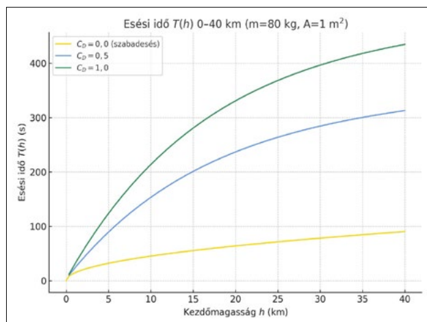
2. ábra. Esési idő a kezdőmagasság függvényében, C_D = 0; 0,5 és 1,0 ellenállási tényezőkkel számolva. A C_D = 0 eset a közegellenállás nélküli szabadesés. A valós adatokhoz a C_D = 0,5 ellenállási tényező áll közel. A számoláshoz használt ugró tömege m = 80 kg, a homlokfelülete A = 1 m 2
