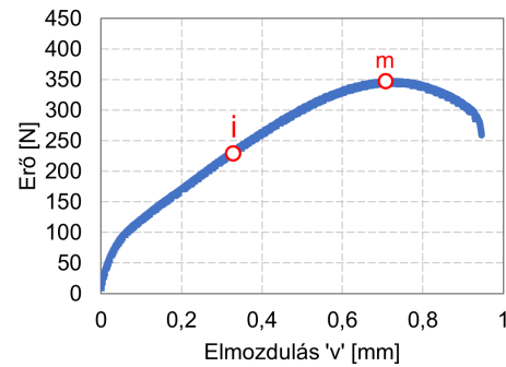
6. ábra: Egy a vizsgált alapanyagokra jellemző erő-elmozdulás diagram
