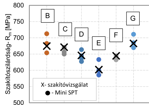
9. ábra: Az új \beta_{R_m} együtthatóval számított szakítószilárdságok összevetése a mini szakítóval meghatározottakkal
