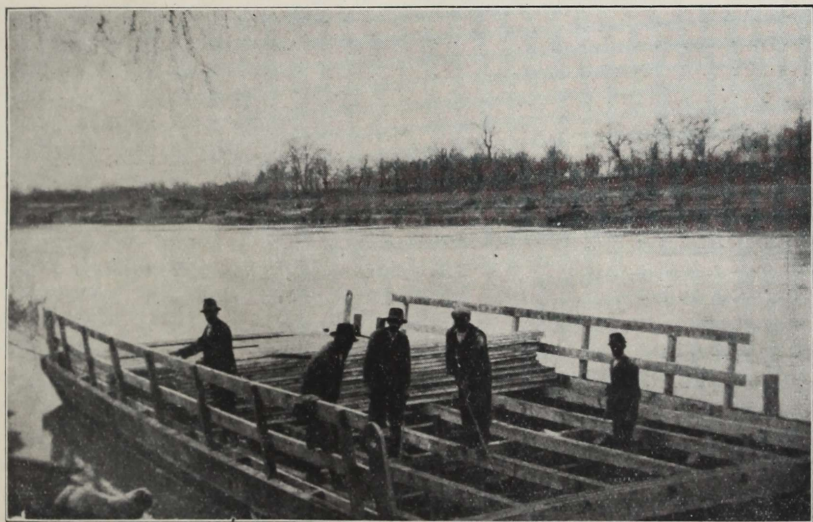
2. A Szamosra csúsztatott, Szamossályi részére készült új hidas belső alkatrészeinek kátrányozása. (Fot. Sőregi J. 1942 április 23.)
