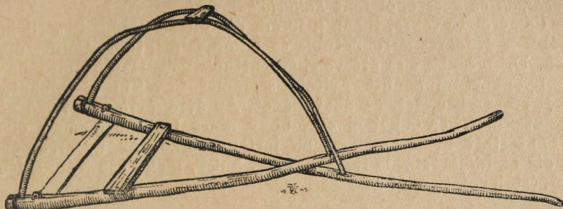
5. kép. Nádvágó (toló) a biharmegyei érkeserői lápokról. H. 333 cm. sz. 60 cm. Déri Múzeum néprajzi osztályában.
