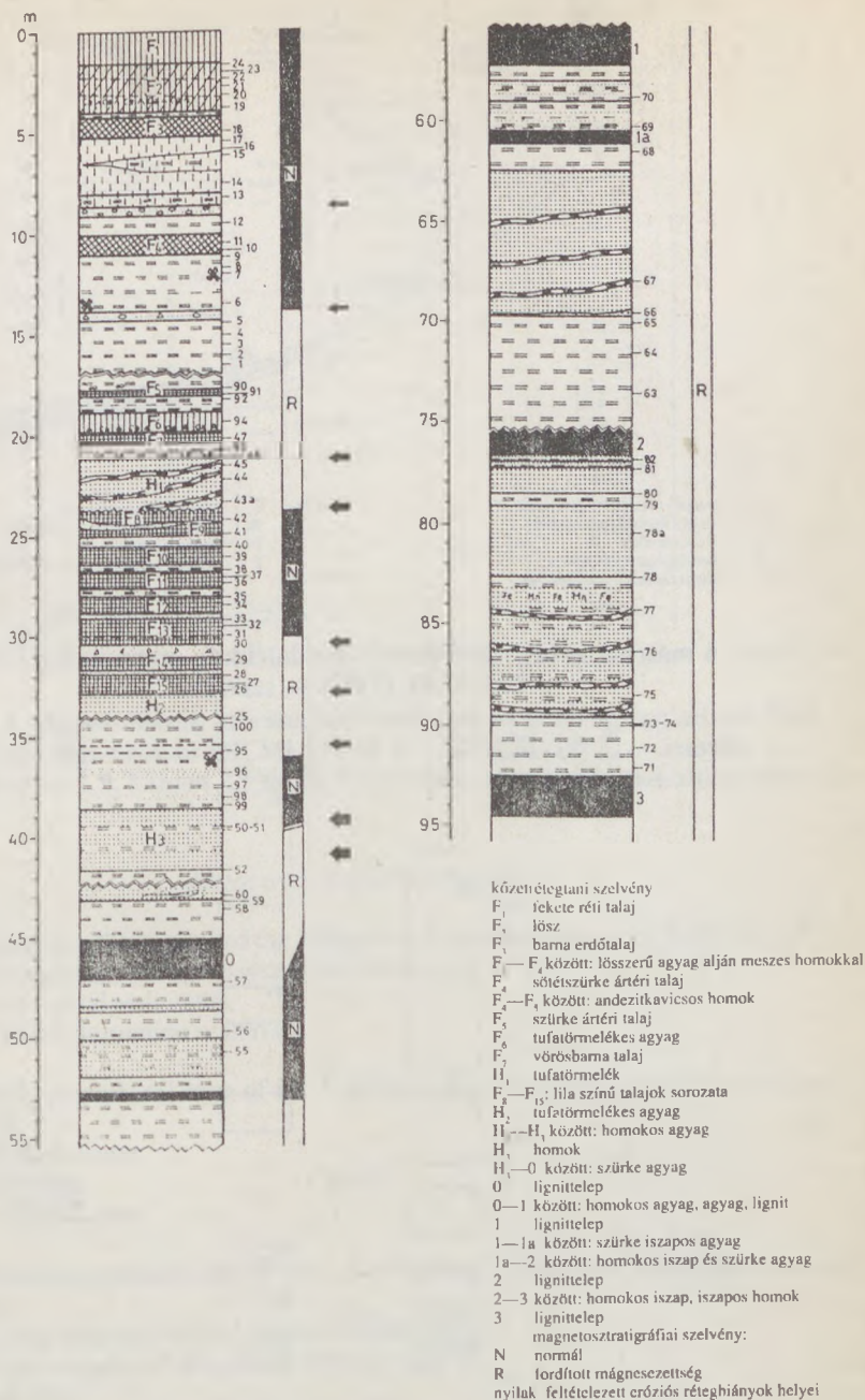
10. ábra: A visontai külszíni lignitbánya összesített szelvénye és a rétegek mágnesessége KRETZOI M. et al (1982) — szerint.
