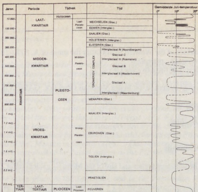
13. ábra: A negyedidőszak időrétegtani beosztása és az eddig regisztrált főbb éghajlati ingadozások DE MULDER E. F. J. et al (1983) — szerint. (Az összesítés nem 1,9, hanem 2,5 millió évnél vonja meg a plio-pleisztocén határt.)
