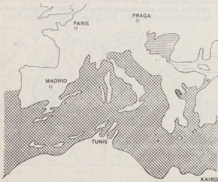
9. ábra: A Pannon-tó ösföldrajzi környezete VELITZELOS E.—GREGOR H. J. (1987) — szerint.
