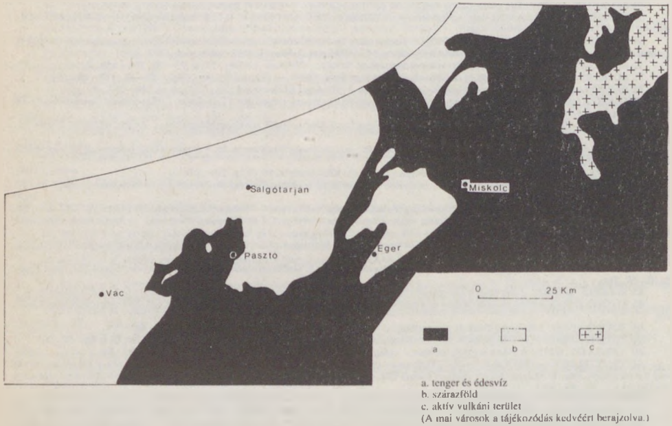
2. ábra: Észak-Magyarország ösföldrajzi térképe a szarmata idején (HÁMOR G. 1985 — nyomán egyszerűsítve).
