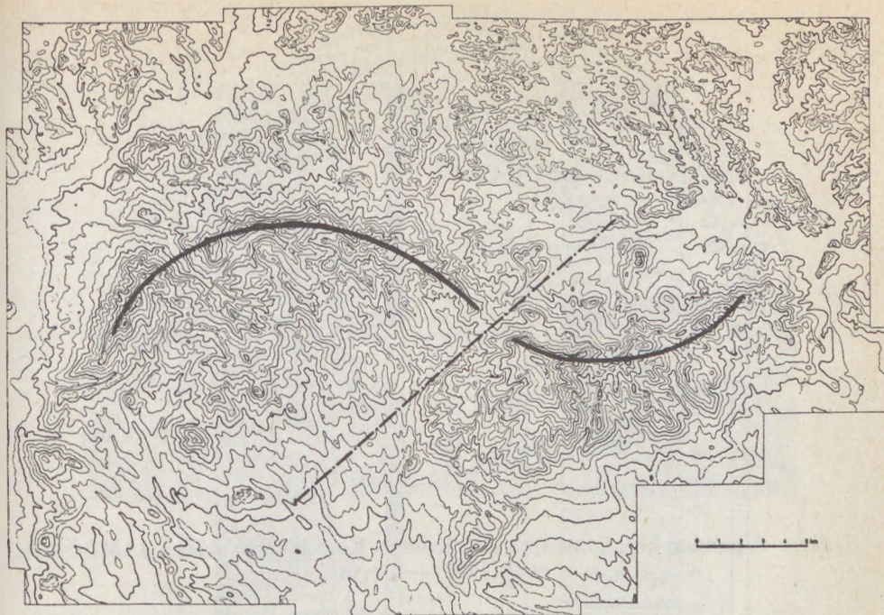
6. ábra: Feltételezett kalderaívek és az eltolódás nyomvonala BALLA Z.—HAVAS L. (1982) — szerint a Mátra szintvonalas térképén. (A Mátra hegység turistatérképe, Kartográfiai Vállalat, 1976, Bp. , alapszintvonalak 50 m-ként.)
