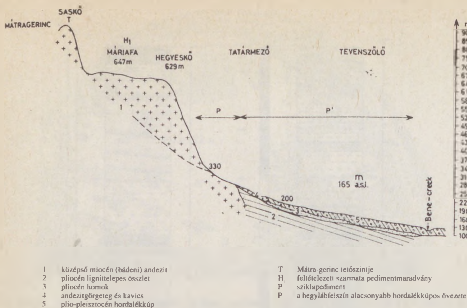
11. ábra: A mátraaljai hegyláb felszín és hordalékkúp metszete KRETZOI M.— PÉCSI M. (1982) — szerint.
