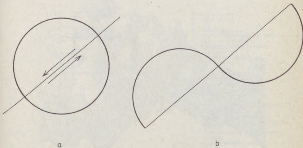
7. ábra: A BALLA Z.—HAVAS L. (1982) — által feltételezett mátrai eltolódás sémája
