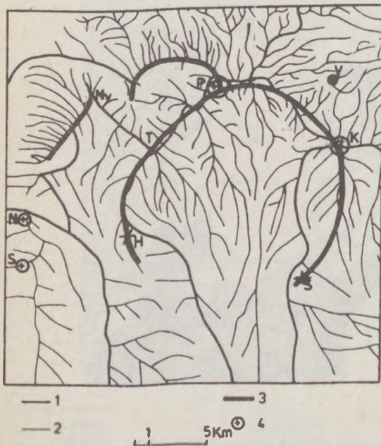
5. ábra: A Mátészalka vízválasztó hálózata GÁBRIS GY. in. SZÉKELY A. (1985) — szerint.
