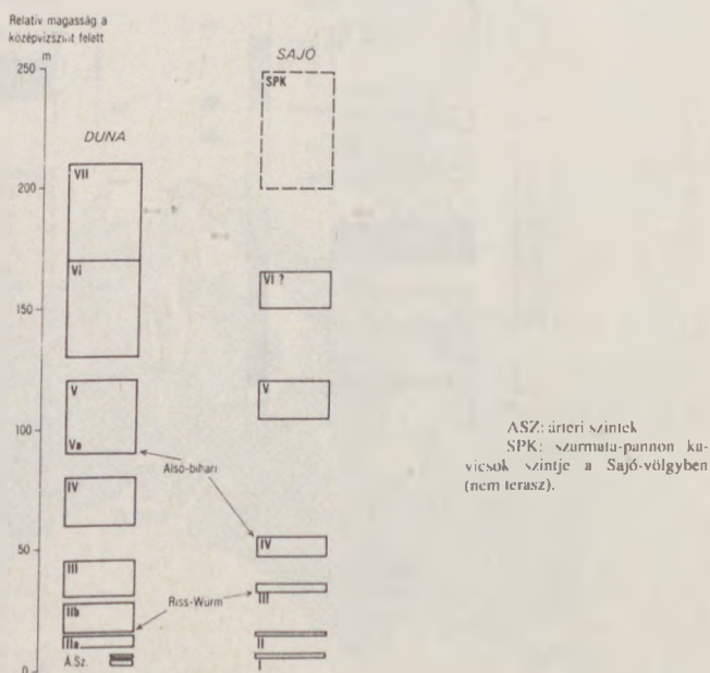
12. ábra: A Duna és a Sajó teraszainak jellemző magassági értékei és ősmaradványokkal bizonyított korrelációja (HIR J. 1989 a).
