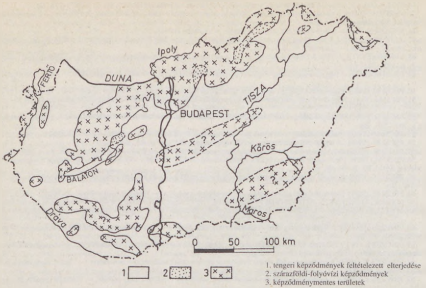
1. ábra: A magyarországi szarmata képződmények ösföldrajzi vázlata JÁMBOR Á. (1971) — szerint.
