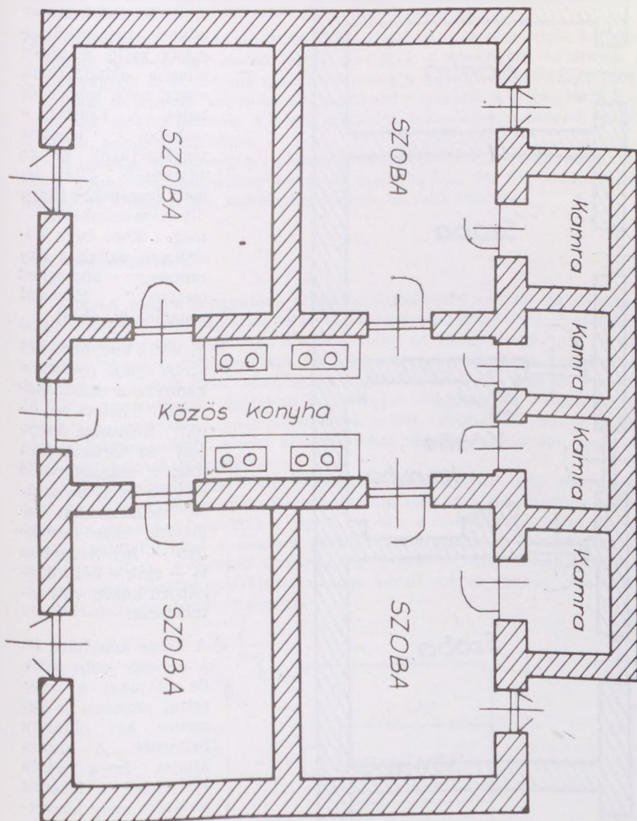
2. ábra. 4 lakásos cselédház. Herencsény
