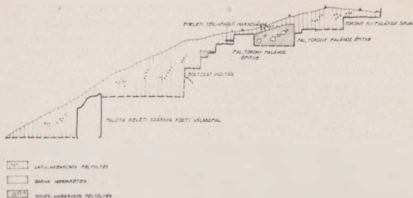
9. kép A palota keleti szárnyában készült észak-déli irányú metszetrajz
