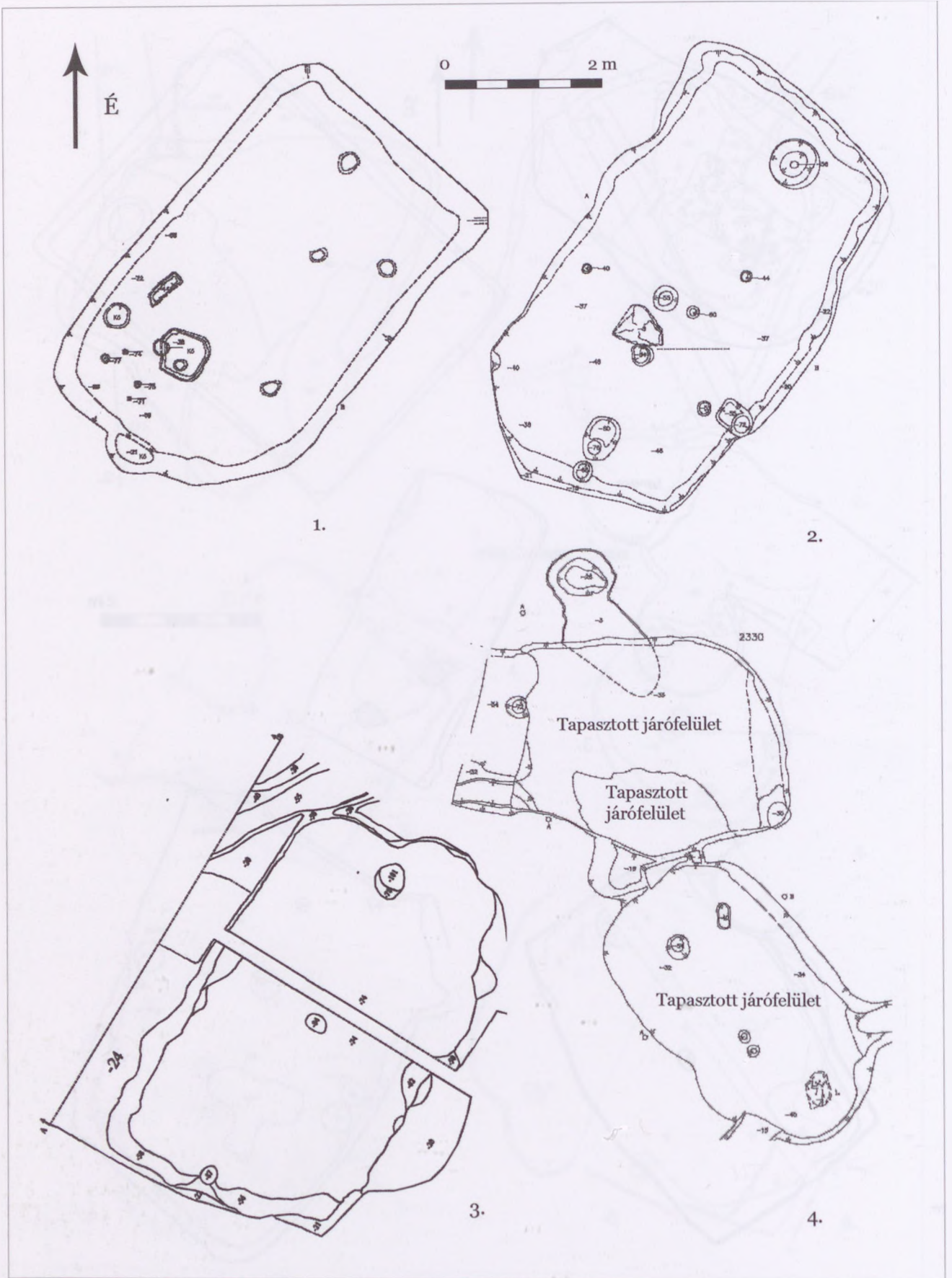
8. tábla: Téglalap alakú házak három cölöppel. 1: 1045. ház; 2: 1026. objektum; 3: 330. objektum; 4: 2330-2331. objektum
