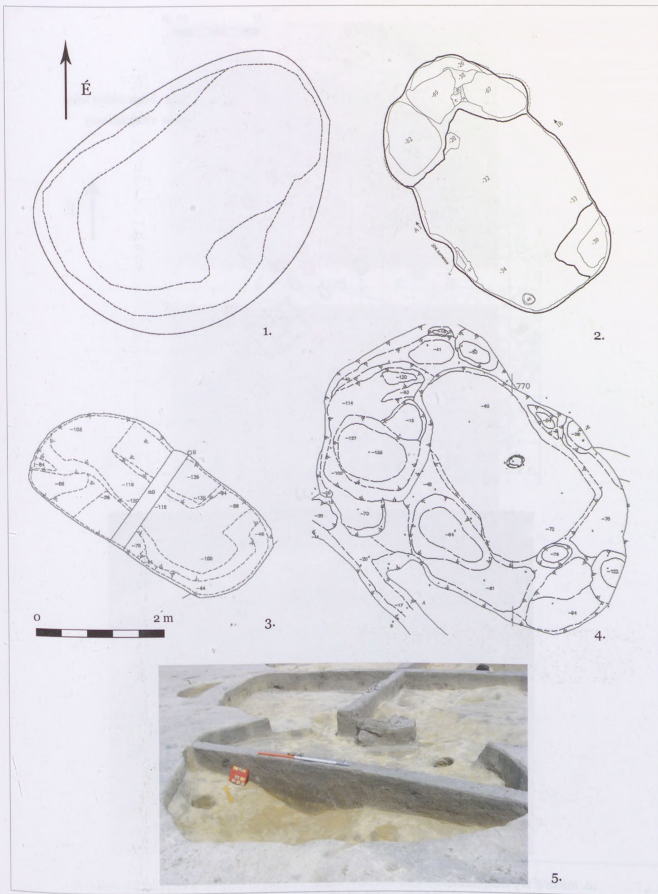
9. tábla: Ovális házak/műhelyek. 1: 280. objektum; 2: 205. objektum; 3: 1052. objektum; 4: 770. objektum; 5: 511. objektum
