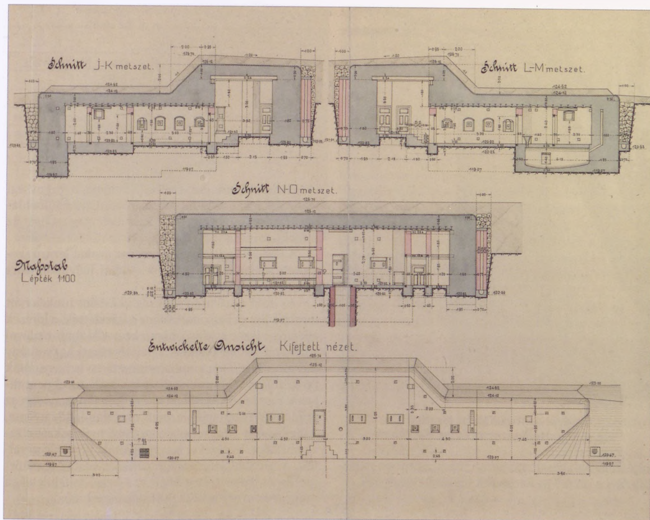
3. kép: A kiserőd metszetrajza és a homlokzat rajza (1909, HM HIM, Térképtár)
