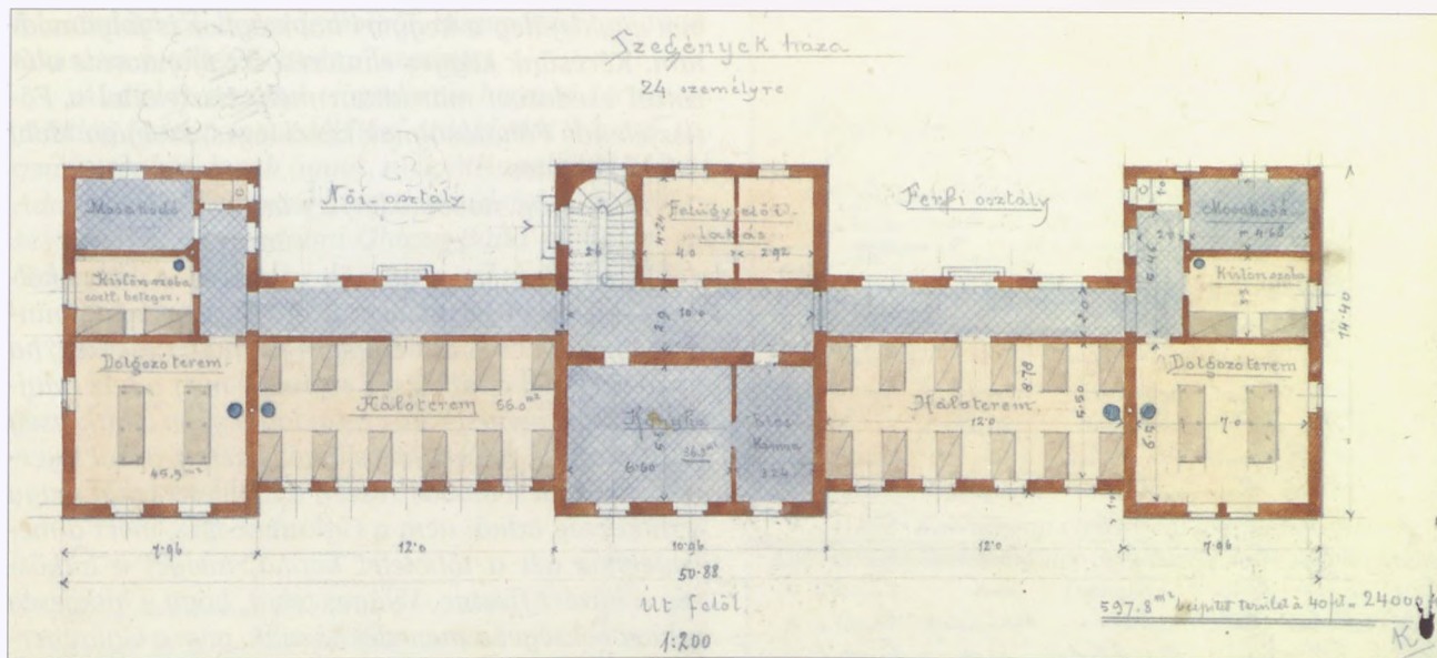
6. kép: A szegények házának tervezett alaprajza (1903)
