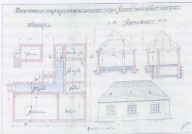
2. A „Miklós-Ferenc” menedékház tervrajza (1902) Abb. 2: Grundriss des „Nicholaus-Franz”-Schutzhauses (1902)
