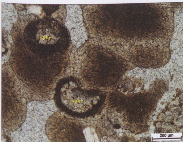
11. kép: Mikrolitokból álló szferolitos (sphe) alapanyag (40/1, 1N)
