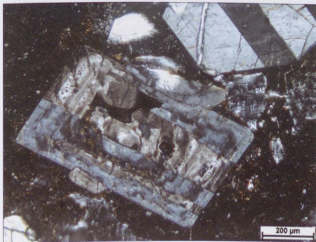
13. kép: Zónás plagioklász (40/1, +N)
