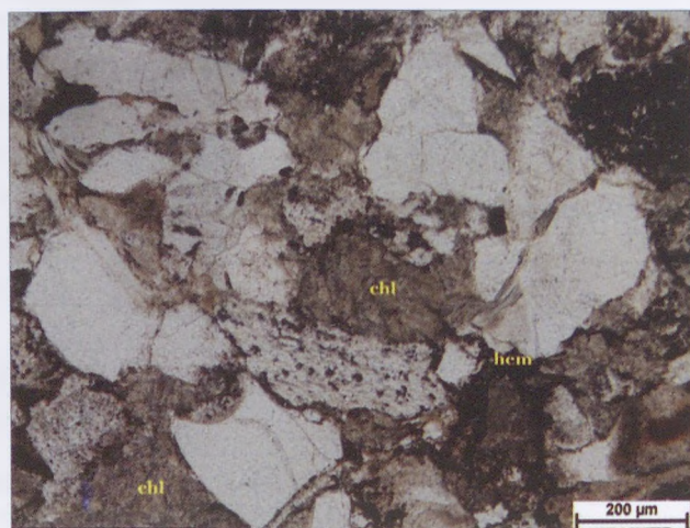
1. kép: Hematitos (hem) és kloritos (chl) kötőanyagú homokkő (25/1, 1N)
