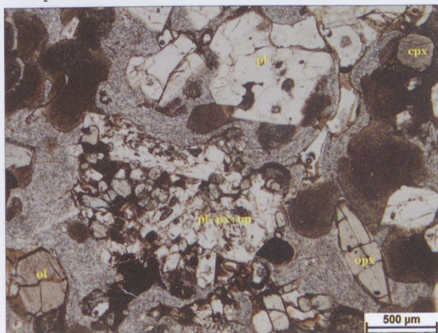
15. kép: Plagioklász, piroxénból és opakásványból álló aggregátum (pl+px+op), olivin (ol), plagioklász (pl), klinopiroxén (cpx), ortopiroxén (opx) (40/1, 1N)
