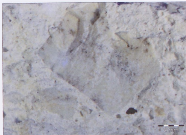
1. kép: A habarcsminta frissen tört felületének mikroszkópos szöveti képe 12x-es nagyítással, ahol különböző méretű törtkövek és a mész kötőanyag látható Abb. 1: Die frische Oberfläche der Mörtelprobe
