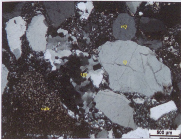
5. kép: Felzites vulkanittörmelék (vulc), jól kerekített kvarc (rQ), monokvarc (Q) és polikvarc (Qp) (25/2, +N)
