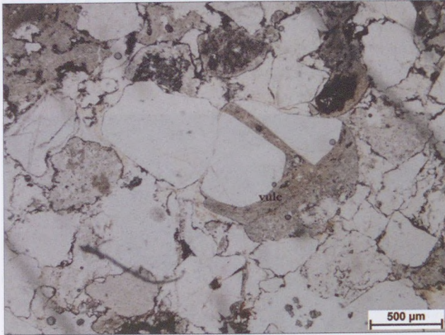
6. kép: Kvarc porfíros savanyú vulkanitszemcse (vulc) (54/1, 1N)
