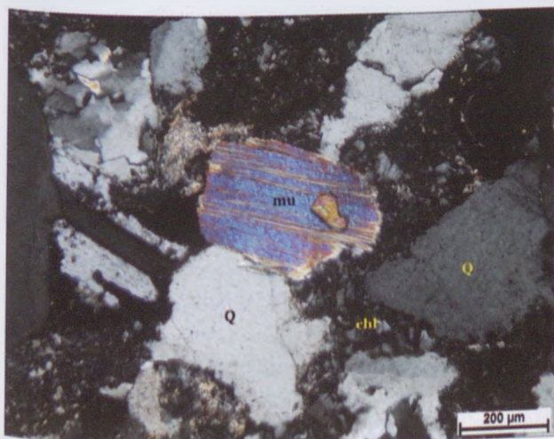
3. kép: Törmelékes eredetű muszkovit (mu), monokvarc (Q) és kloritos kötőanyag (chl) (13/2, +N)
