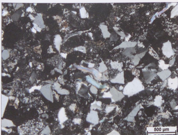
10. kép: Jól osztályozott homokkő általános szöveti képe (13/1, +N)
