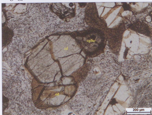
14. kép: Sajátalakú olivin kristályok (ol) és szferolit (sphe) (40/1, 1N)
