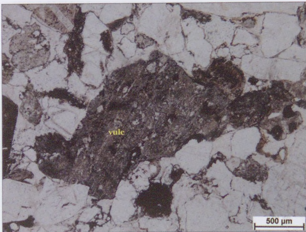
7. kép: Folyásos szövetű vulkanittörmelék (vulc) (25/2, 1N)
