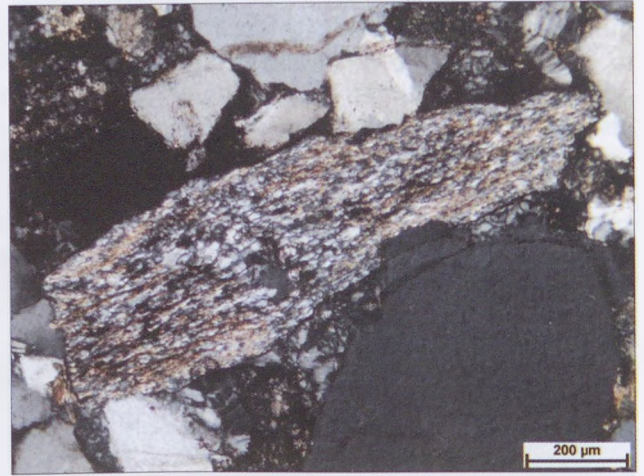
8. kép: Foliált szövetű metamorf kőzettörmelék (25/4, +N)
