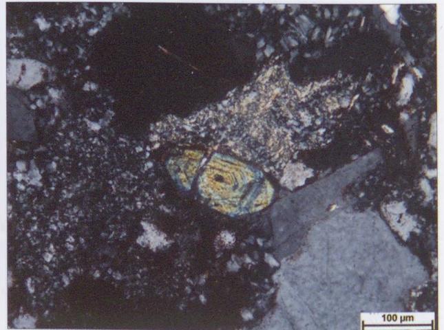
9. kép: Zónás cirkon (középen) (13/1, +N)
