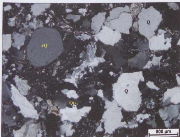
2. kép: A kvarc változatai: jól kerekített kvarc (rQ), monokvarc (Q) és polikvarc (Qp) (13/2, +N)
