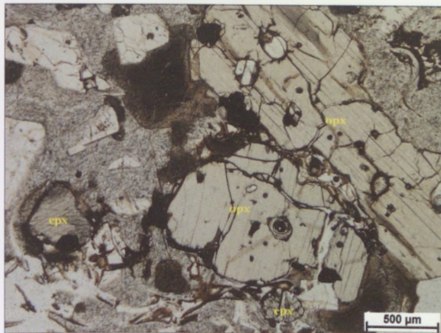
12. kép: Sajátalakú piroxén fenokristályok: klinopiroxén (cpx), ortopiroxén (opx) (40/1, 1N)
