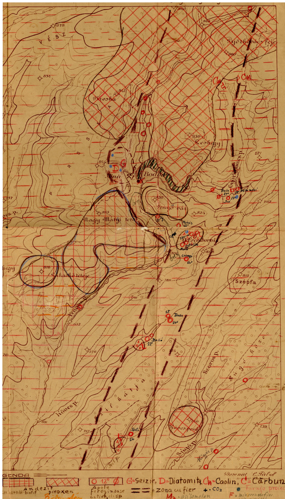
3. ábra Bodvajbánya (Magyarhermány) geológiai térképázata (a vajdahunyadi vasvárnak készített dokumentáció térkép alapján)
