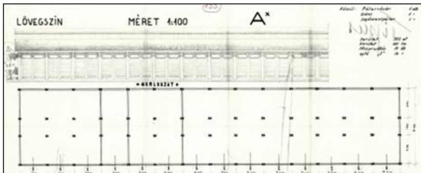
6. ábra C. típusú lövegcsin látképe és alaprajza Forrás Hadtörténelmi Levéltár
