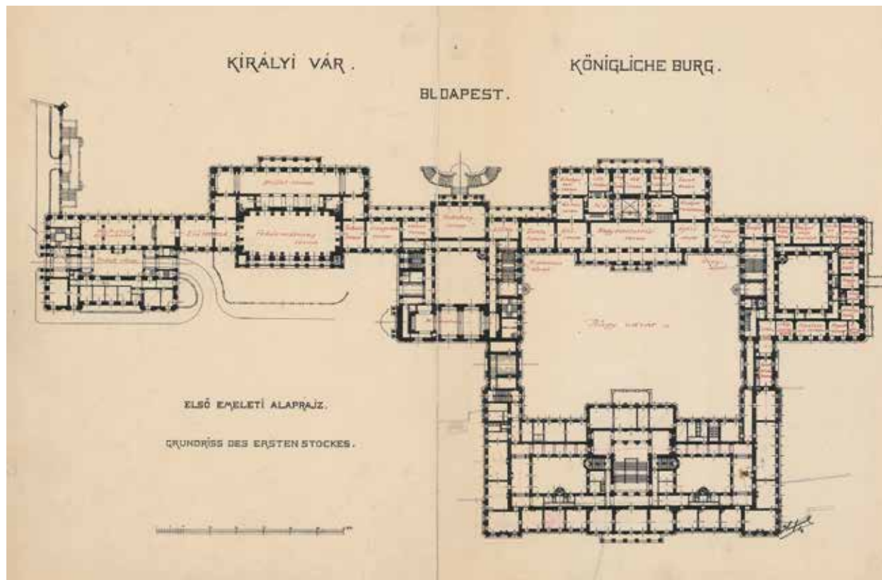
83. A budai királyi palota első emeleti alaprajza a kibővítés után, a terembeosztást jelző 1940 körüli (piros) feliratokkal Budapest, Budapesti Történeti Múzeum, Kiscelli Múzeum, Építészeti Gyűjtemény, ltsz. 304
