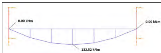
4. ábra. Egy csuklós kapcsolat hajlítónyomaték-diagramja
