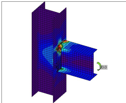
2. ábra. A vizsgált kapcsolat végeselem-modellje
