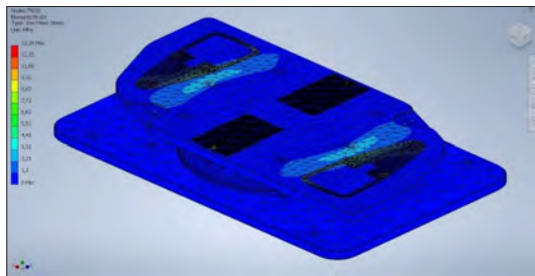
8. ábra. A redukált feszültség szemléltetése [2]
