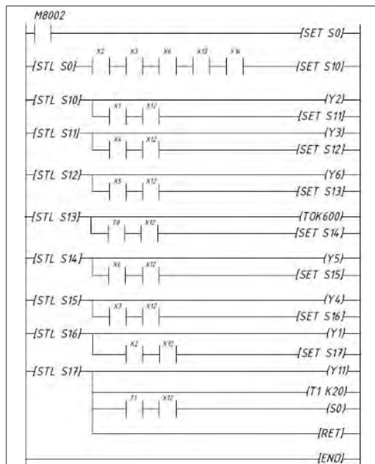
18. ábra. Létradiagram [2]
