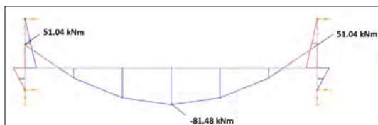
3. ábra. A vizsgált kapcsolat hajlítónyomaték-diagramja
