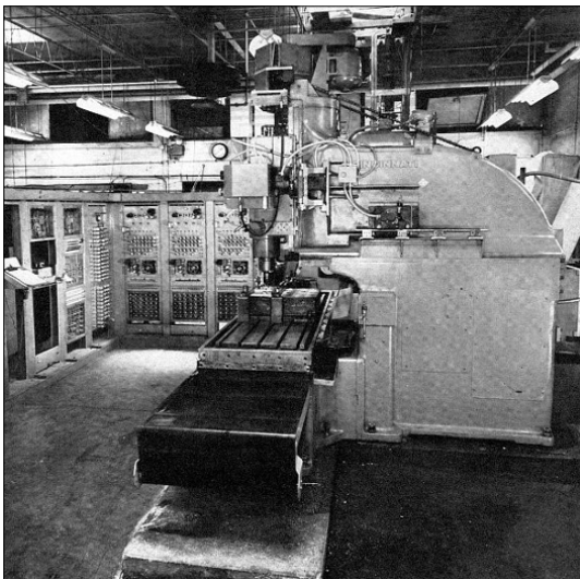
2. ábra. Az első NC-marógép (Cincinnati Milacron Hydrotel)
