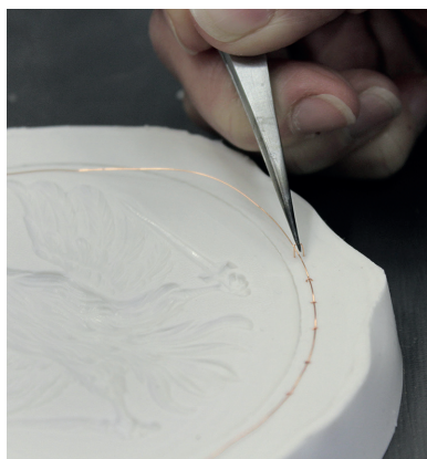
10. „U” alakú tűkkel a vékony rézdrót rögzítése a minta köré.
