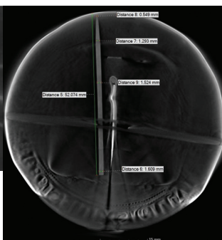
19. kép – A pecsét CT metszeti képe. A belső szerkezetben detektáltunk egy hengeres komponenst, melynek hossza ~ 52 mm, átmérője ~1.6 mm. A komponens az egyik végpontjában kúpos kialakítású, anyaga feltehetően a „rugós” lemez anyagával megegyező.
