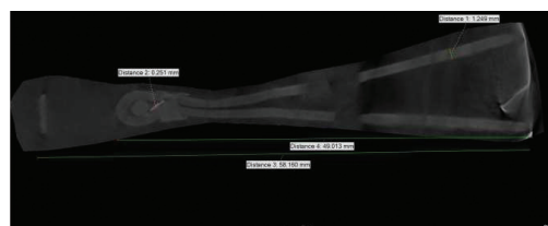
25. kép – CT metszeti kép – Rögzítőszegek geometriai méretei. A „Distance 2”-vel jelölt lemez más anyagminőséggel készült, mint az rögzítőszegek többi eleme.
