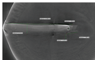
34. kép – CT metszeti kép – az árárszeg geometriai adatai. A pecsét belsejében detektáltunk egy ~ 4,3×7,4 mm befoglaló méretű 1mm-nél kisebb falvastagságú derékszögű lemezt.
