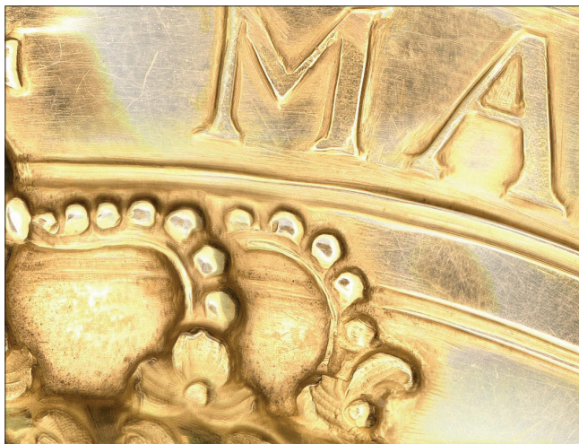
76. kép – Öntésre utaló felületi porozitás nyomai
