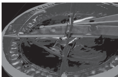
20. kép – A pecsét CT metszeti képe. A röntgen felvételnél (15. kép) jelöltük a lemezes elemek jelenlétét. A CT metszeti képek elemzése során a felvételeken porozitást (fekete foltok) detektáltunk, az adott szegmensben hőhatással járó beavatkozás (pl. javítás, pótlás) érte a pecsétet.
