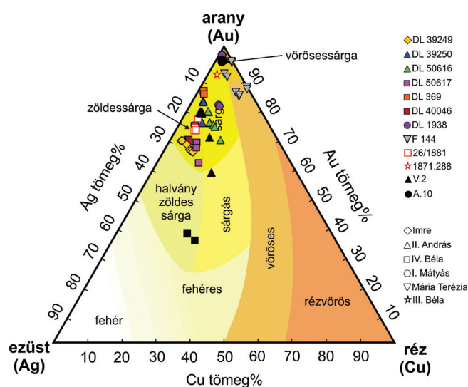
1. ábra: A vizsgált aranybullák kémiai összetétele a hXRF mérések alapján az Au–Ag–Cu háromszögdiagramon ábrázolva.
