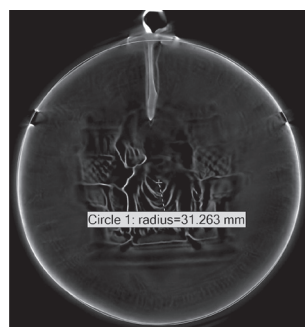
2. kép – CT metszeti kép – Pecsét átmérő ~ 62,5 mm
