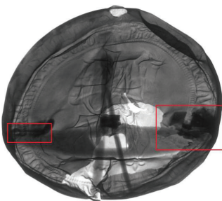
27. kép – Pecsét röntgen képe – A vizsgált pecsétek közül ez a belső kialakításában a legváltozatosabb. Kereszt irányú merevítő csakúgy mint a „369”-es pecsétnél, nem a legnagyobb keresztmetszetben, hanem az átmérő 2/3-ánál helyezkedik el. A merevítő közepén szintén van egy trapéz alakú kivágás, amin átmegy a merevítőre merőleges irányban az rögzítőszegeg. Ennél a pecsétnél is jelentős a hozzáadott (esetleg a pecsét alkotásánál is már használt) javítási anyag. Különbség, hogy ennél a pecsétnél detektáltunk egy „U” alakban hajlított vékony lemezt, amely jelenléte sem a merevítést, sem a javítást nem indokolja (1)-el jelölt elem.
