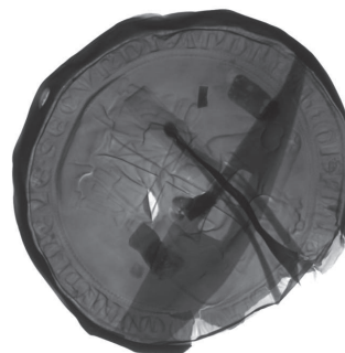
22. kép – A pecsét röntgen képe – A kereszt irányú merevítő nem a legnagyobb átmérőben, hanem annak kétharmad részénél helyezkedik el. Közepén egy négyszög alakú kivágás, ebben megy át a merevítésre merőleges irányú rögzítőszegeg. Feltételezhető, hogy a merevítésnél utólagos javítás is történt – a bal oldali forrasztás egyenes vonalú, míg a bal oldali jelölt szegmensben nagyobb területen detektáltunk porozitást, apróbb lukakereket.
