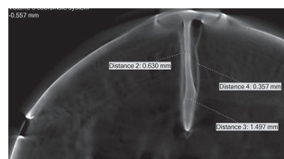
4. kép – CT metszeti kép – geometriai méretek. A kisebb falvastagságú lemez más anyagminőség, mint a középső, vastagabb szegmens.
