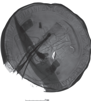
29. kép – Pecsét röntgen képe
