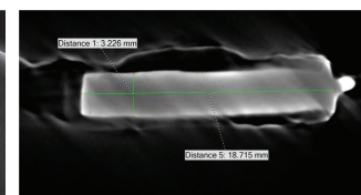
5. kép – CT metszeti kép – A rögzítőszeg geometriai méretei
