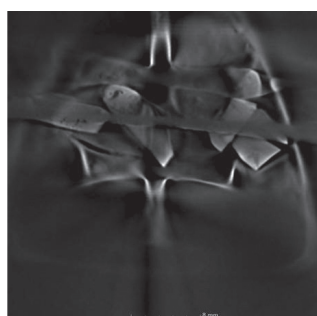
20. kép – A pecsét CT metszeti képe. A röntgen felvételnél (15. kép) jelöltük a lemezes elemek jelenlétét. A CT metszeti képek elemzése során a felvételeken porozitást (fekete foltok) detektáltunk, az adott szegmensben hőhatással járó beavatkozás (pl. javítás, pótlás) érte a pecsétet.
