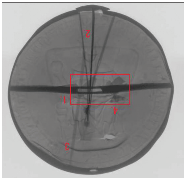
37. kép – A belső szerkezet CT felvétele, pirossal jelölve a forrasztás nyomait
