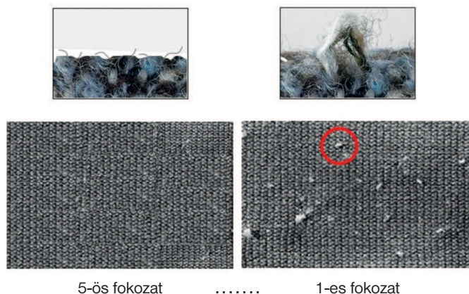
3. ábra. Értékelő etalonok a száلكihúzóási hajlam buzogányos vizsgálatához
