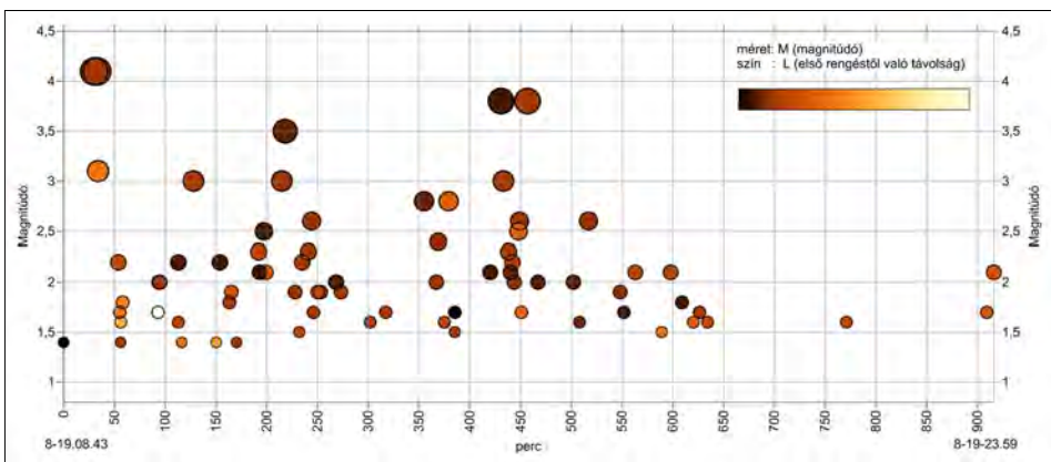
4. ábra | Békési rengések, utórengések, rengésrajok – időrendi sorrendben, méret a magnitúdo szerint, szín a (0–7 km) távolság szerint (augusztus 19-én 8.00–24.00 óra között)
