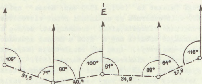
7. kép: Tájéolós sokszögelés
