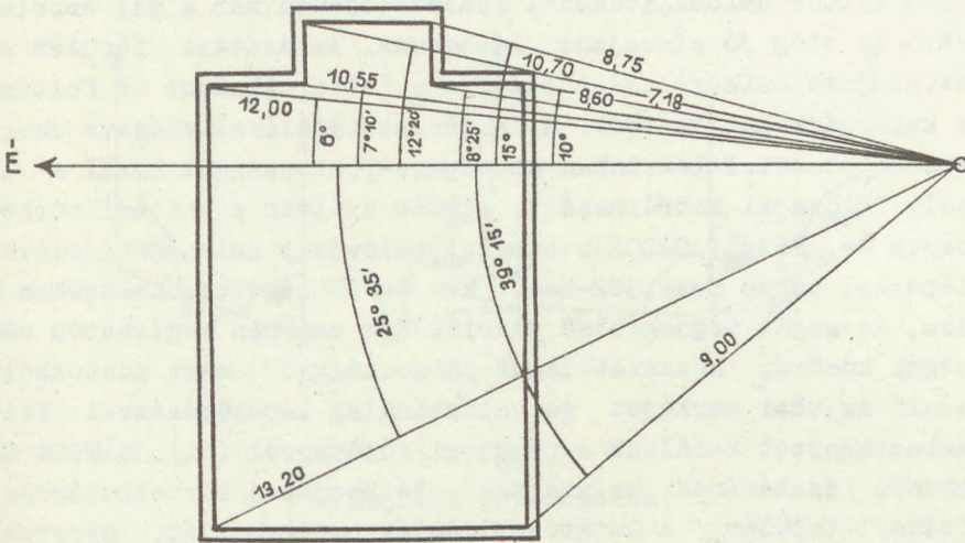
6. kép: Poláris koordinátamérés
