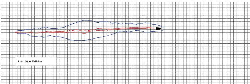
17. kép: Keréklakatos pisztolyból kilőtt golyó, hasáblövedék és modern 9 mm-es Luger lőszer hatása ballisztikai zselatinban. Piros: maradandó sebcsatorna, kék: az időszakos sebcsatorna kialakulásának külső határa, 1 négyzet = 1 \times 1 cm
