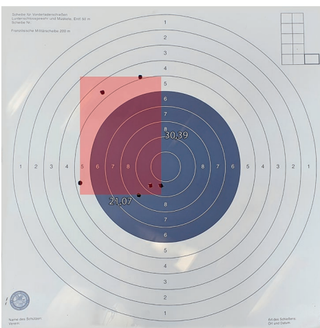
15. kép: A keréklakatos pisztoly szórásképe 25 m-en gömblövedékkel
