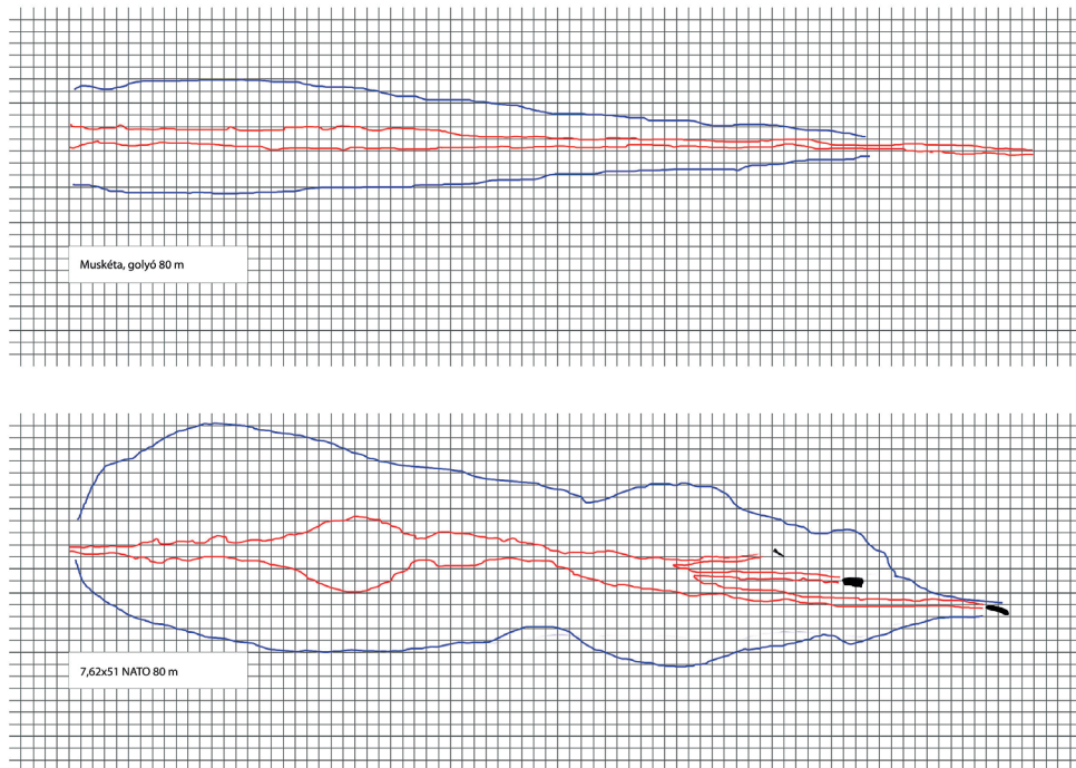
11. kép: Muskétagolyó és .308 Win lőszer hatása ballisztikai zselatinban. Piros: maradandó sebcsatorna, kék: az időszakos sebcsatorna kialakulásának külső határa, 1 négyzet = 1 × 1 cm
