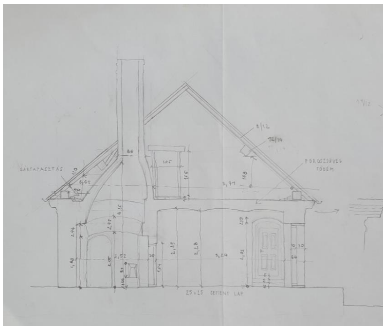
Hidegkúti parasztház metszete (Schlögler Dóra manuáléja)
