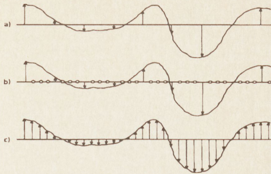
1. ábra. A túlmintavételezés technikája négyszeres túlmintavételezés esetén. a) Az analóg és a mintavételezett jel; b) A négyszeres túlmintavételezett jel a zérus amplitúdójú mintákkal; c) A sávhatárolt túlmintavételezett jel
