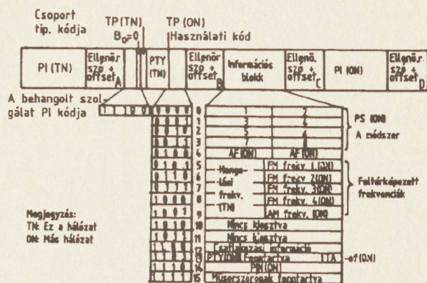
3. ábra. Bővített információ más hálózatokról (EON) – 14A csoport típus
