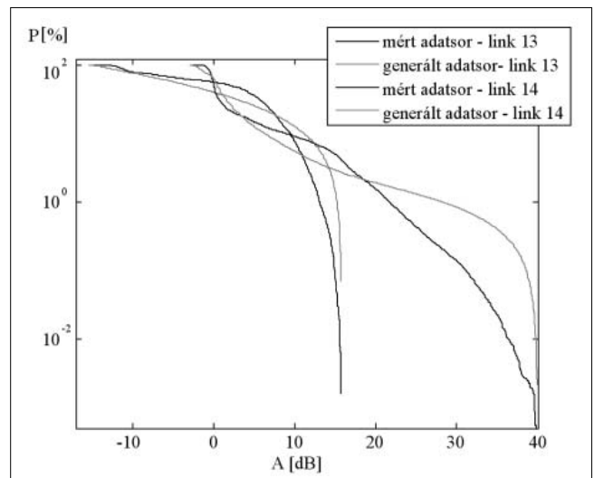
2. Táblázat A Gaussi fade slope modell paraméterei
