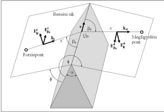
5/b. ábra A diffrakció koordinátarendszere
