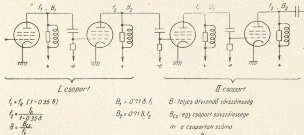
22. ábra. Lépcsős hangolósú erősítő, kétlépcsős csoportok
