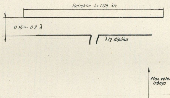
10. ábra. Reflektor alkalmazása
