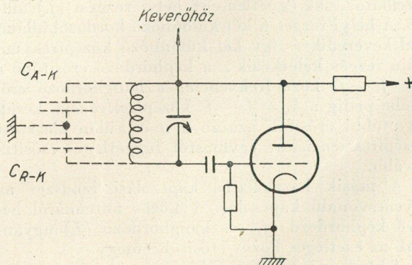
19. ábra. Ultraudion rendszerű oszillátor
