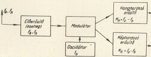
12. ábra. Transzponáló rendszerű vevőkészülék vázlatos elrendezése
