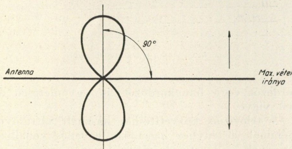
8. ábra. Félhullámú dipólus vázlatos polárdiagrammja
