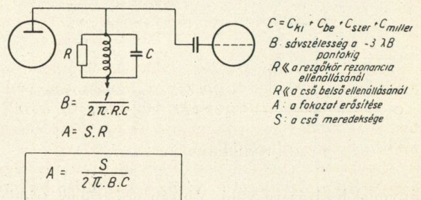
14. ábra. Egyes rezgőkör jellemző adatai
