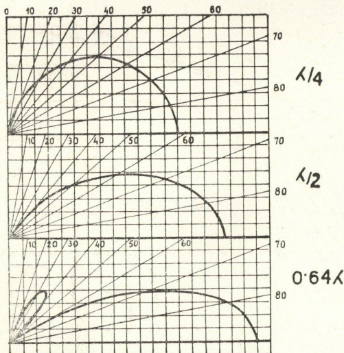
Különböző antennák vertikális polárisdiagramja abszolút jó föld esetén.
