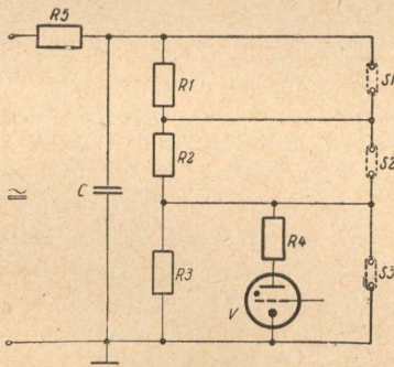
2. ábra. Villanó megvilágító rendszer három villanócső egyidejű működtetéséhez.
