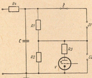
4. ábra. Villanó megvilágító rendszer robbanóhuzalokkal való megvilágításhoz. C = kondenzátor, E = robbanóhuzal, R1—R4 = ohmos ellenállások, S1—S2 = szikraközök, V = thyatroncső
