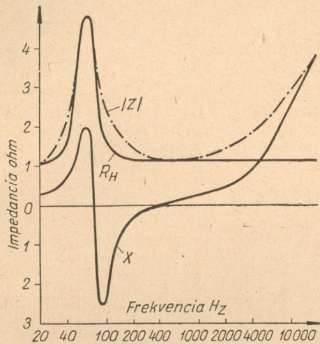
7. ábra. Dinamikus hangszóró impedanciája a frekvencia függvényében. R = a lengőcséve ohmos ellenállása. R_H = a hangszóróimpedancia ohmos összetevője. X = a hangszóróimpedancia képzetes összetevője. |Z| = a hangszóróimpedancia abszolút értéke. (Kinsler—Frey nyomán).*
