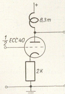
34. ábra. R - L katódkövető kapcsolású differenciátor
