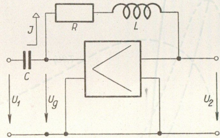
18. ábra. Visszacsatolt erősítőt tartalmazó C—R—L differenciátor
