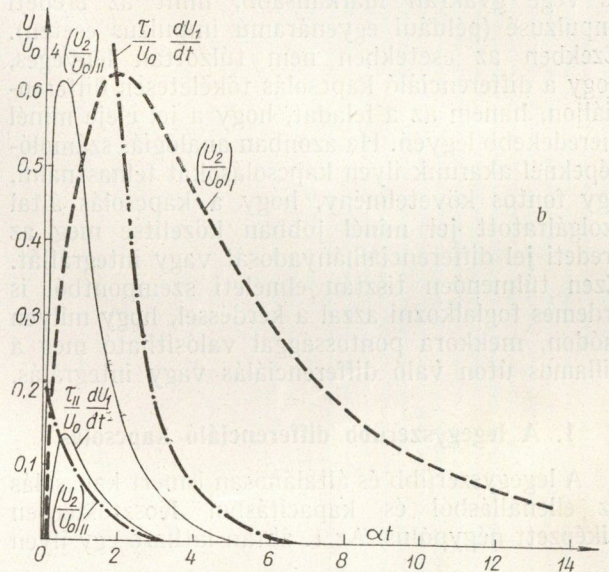
3. ábra Valódi impulzus differenciálása
