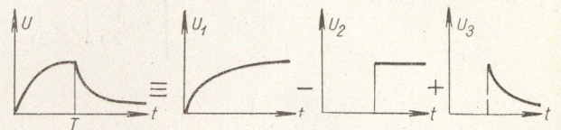
38. ábra. Feszültséggörbe felbontása
