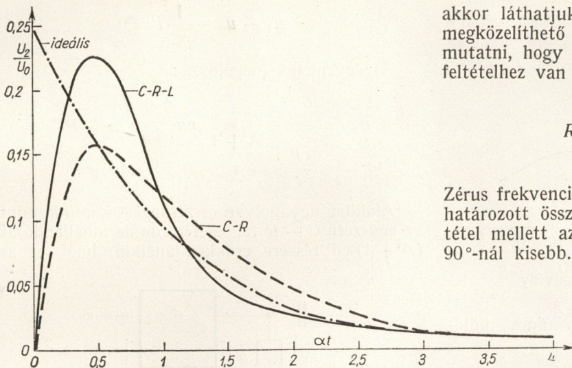
12. ábra. Valódi lökésfeszültség differenciálása C—R és C—R—L differenciátoron - · - · - az ideális derivált \tau -szorososa - - - - C—R differenciátor jele ——— C—R—L differenciátor jele Az ábra az \alpha\tau = 4 esetre vonatkozik
