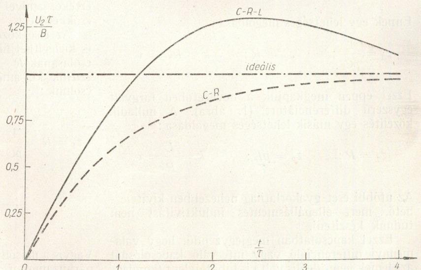
11. ábra. Lineárisan változó feszültség differenciálása C-R és C-R-L differenciátoron - · - · - az ideális derivált \tau -szorosa - - - - C-R differenciátor jele - - - - C-R-L differenciátor jele
