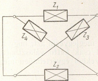
9. ábra. X-tag, mint legáltalánosabb négypólus. A primer oldalról rövidzár a zérus belső ellenállású feszültség-generátort reprezentálja
