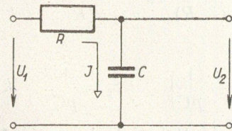
23. ábra. A legegyszerűbb R-C integráló kapcsolás
