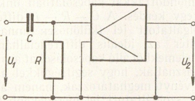
15. ábra. C—R differenciátor láncbakapcsolt erősítővel
