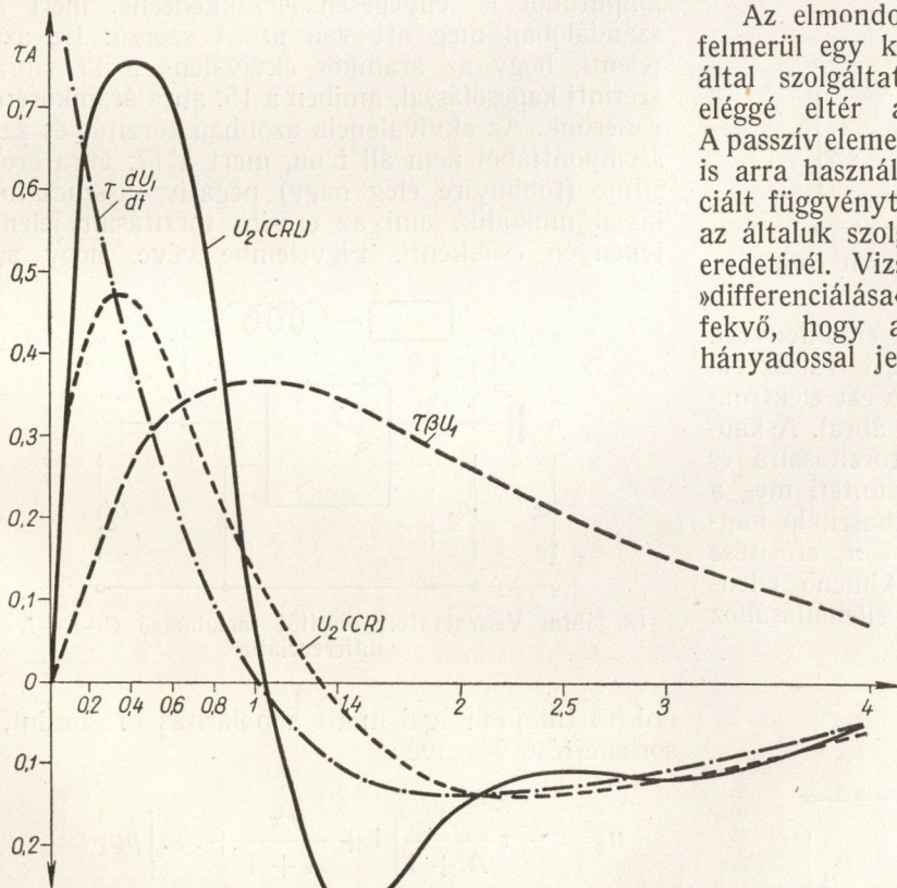
13. ábra. Lapos impulzus differenciálása C—R és C—R—L tagon. U_1 = Ate^{-\beta t} (Ilyen impulzusformával közelíthetők meg például a Geiger—Müller számlálószevek által adott jelek).
