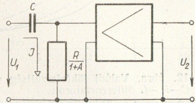
17. ábra. Visszacsatolt erősítőt tartalmazó C—R differenciátor helyettesítő képe
