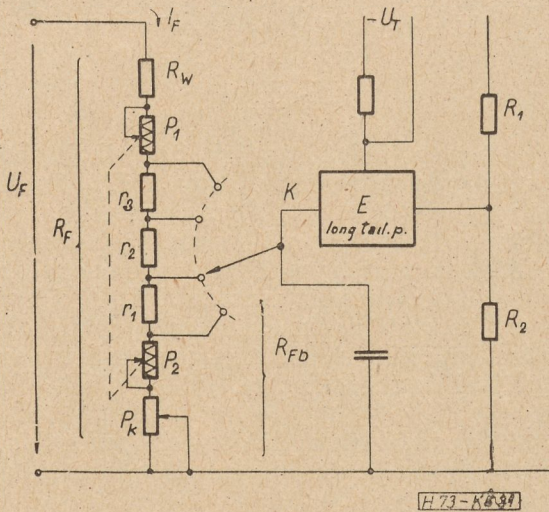
31. ábra. A referencia osztólánc kialakítása
