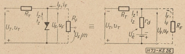
26. ábra. Zener-dióda referenciaforrás és helyettesítő áramkör
