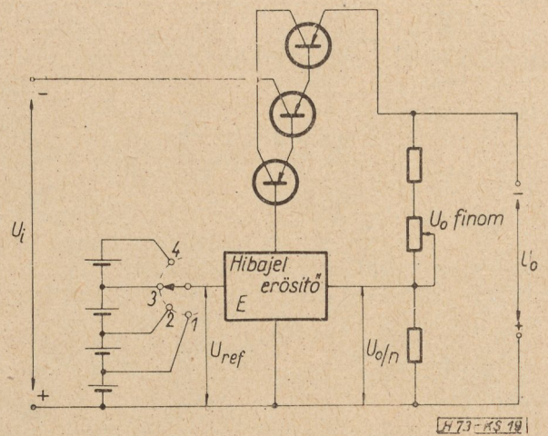
19. ábra. Változó feszültségű telep-referencia stabilizátor
