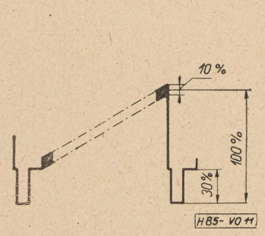
11. ábra. Linearitásméréshez használt jel az adó bemenetén
