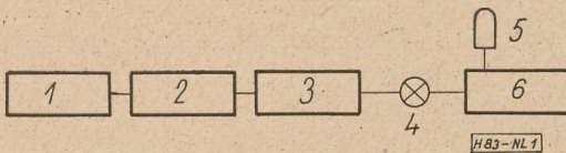
1. ábra. Az ultravákuum előállításának tömbvázlata. 1—elővákuum szivattyú; 2—olajdiffúziós szivattyú; 3—speciális kifagyasztó; 4—ultravákuumszelep; 5—Bayard—Alpert-féle ionizációs mérő; 6—vákuumrendszer
