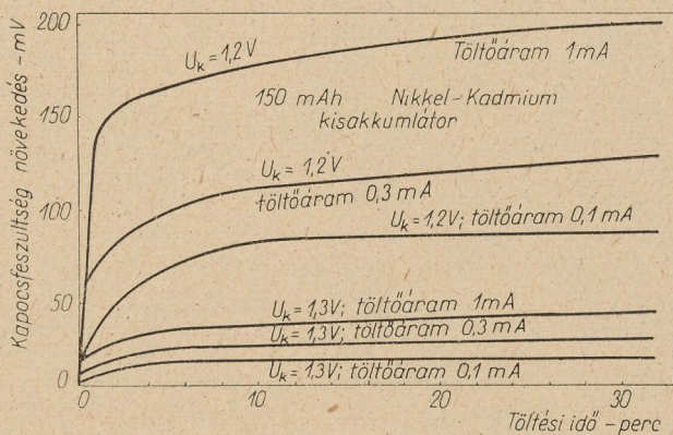
22. ábra. Ni-Cd kisakkumulátor kapocsfeszültség függése a töltőáramtól
