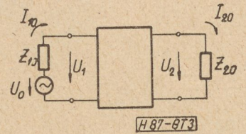
3. ábra. Hullámimpedanciájával lezárt négypólus
