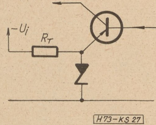
27. ábra. Zener-diódás referencia kisigényű kapcsolásokhoz
