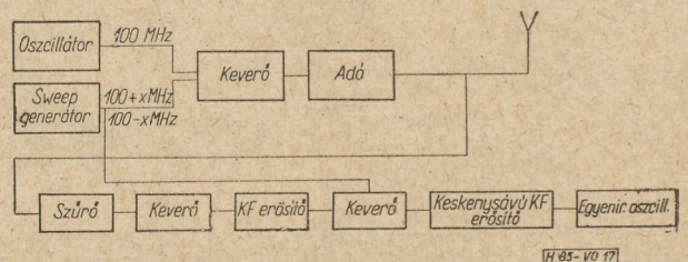
17. ábra. Kétoldalsáv demodulátor tömbvázlata
