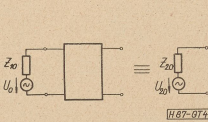
4. ábra. Négypólus szekunder oldalának feszültséghelyettesítő kapcsolása
