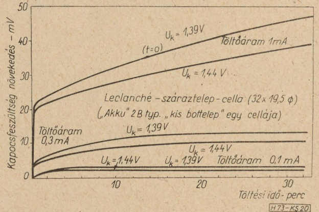
20. ábra. Száraztelep kapocsfeszültség függése a töltő- áramtól
