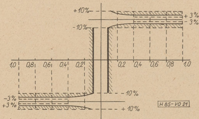
21. ábra. CCIR tűrésdiagram négyszögfeszültség átvitelhez
