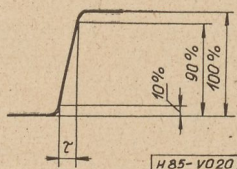
20. ábra. Felfutási idő meghatározása
