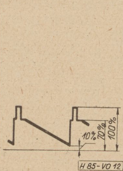
12. ábra. Linearitásméréshez használt jel az adó kimenetén
