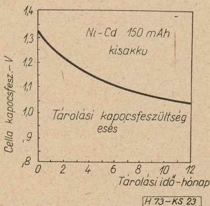
23. ábra. Ni-Cd kisakkumulátor kapocsfeszültségesése
