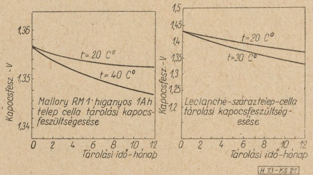
21. ábra. Száraztelepek tárolási kapocsfeszültség- esése
