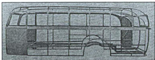
13. ábra AZ AUTÓBUSZSEKRÉNY FÉMVÁZA
