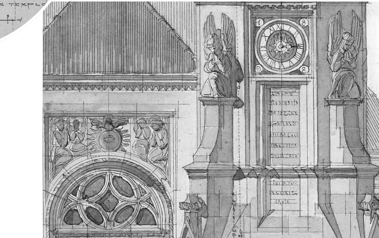
A felsőrönöki Szent Imre-templom tervrajzai, 1898.
