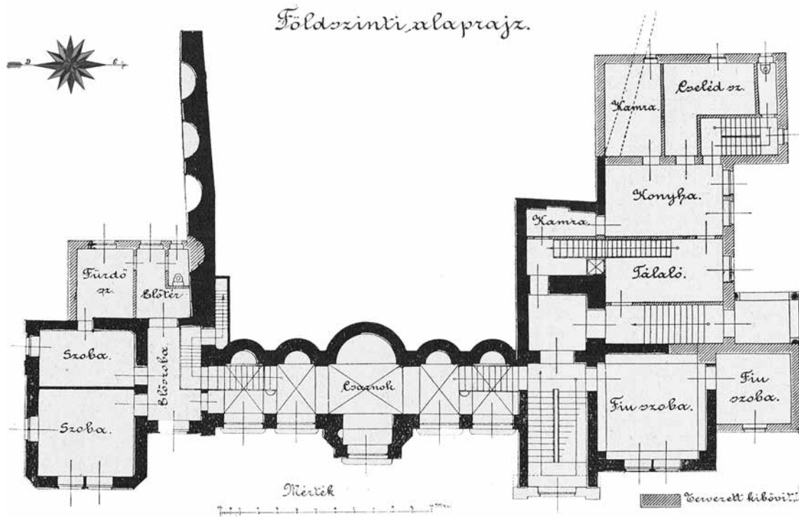
12. kép | Wälder Gyula: A Bagolyvár átépítéséhez készített földszinti alaprajz (Bodányi, 1910. 179. p.)
