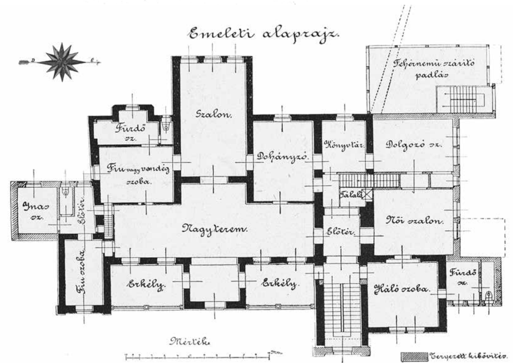
Wälder Gyula: A Bagolyvár átépítéséhez készített emeleti alaprajz (Bodányi, 1910. 180. p.) 13. kép
