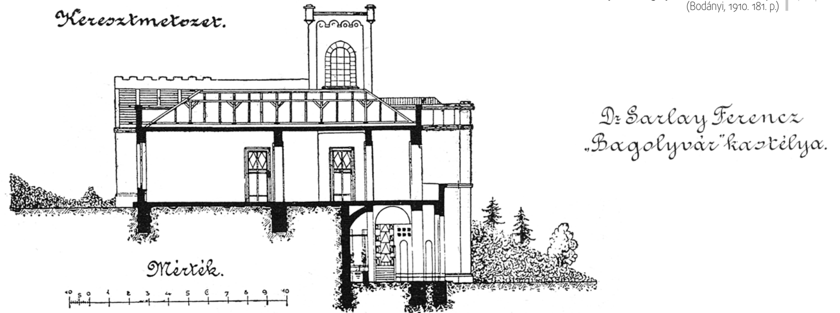
Wälder Gyula: A Bagolyvár keresztmetszeti rajza (Bodányi, 1910. 181. p.) 14. kép
