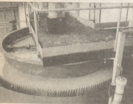
A flotátorban fajsúlykülönbség szerint választják szét az olajos-vizes komponenseket.
